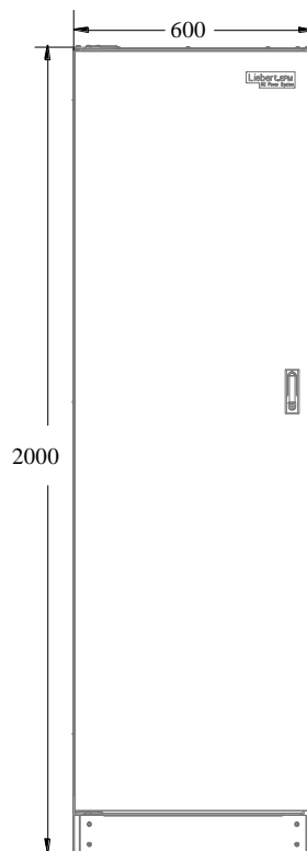
图6-3 电池开关柜正面尺寸（单位：mm）
