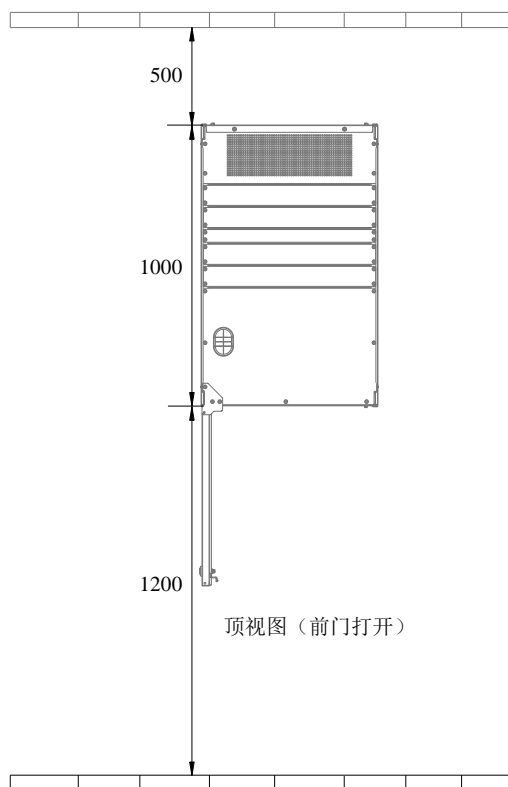
图6-4 电池开关柜空间尺寸 (单位: mm)
