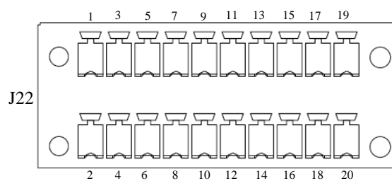
图3-7 干接点接口 J22 示意图
