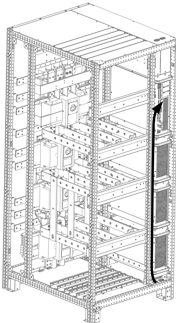
图3-12 600kVA 信号电缆进线示意图（下进线）
