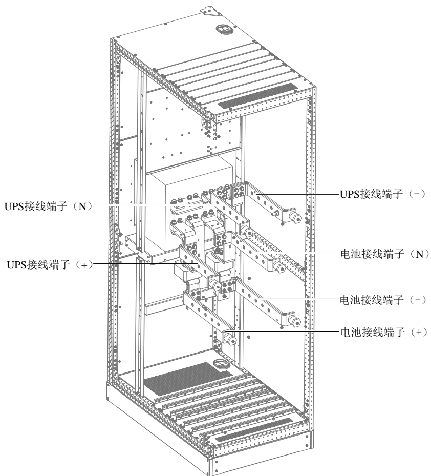
图6-5 总体电池开关柜内部接线端子说明
