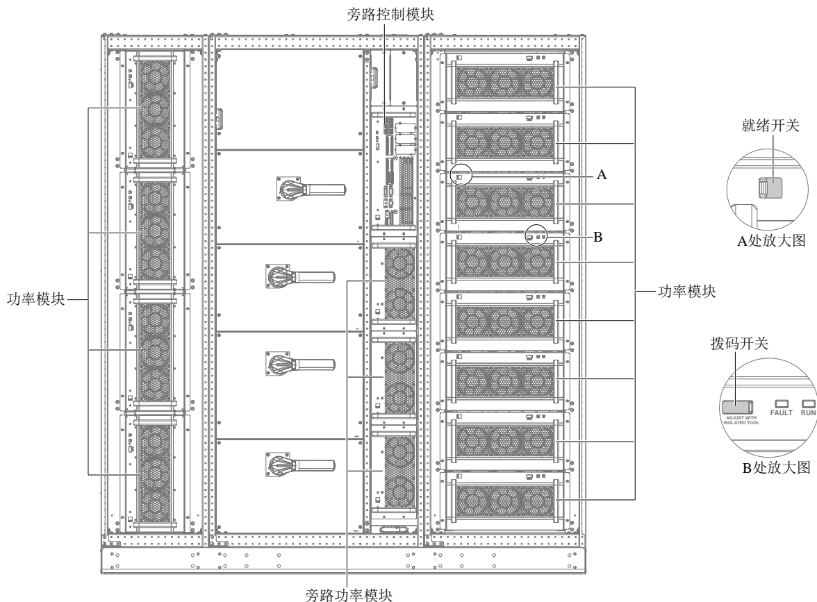
图2-7 600kVA 功率模块安装示意图
