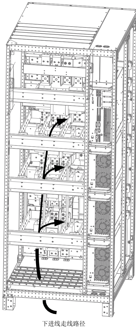
图3-4 600kVA 功率电缆走线示意图（下进线）
