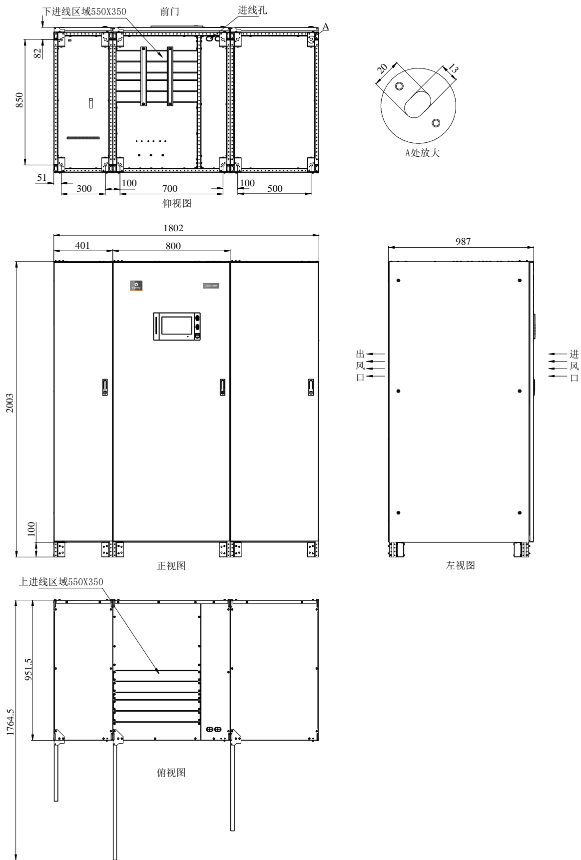
图2-8 600kVA 安装尺寸示意图 (单位: mm)
