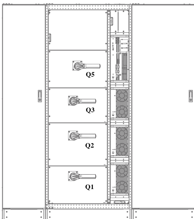
图5-1 UPS 电源开关位置示意图
