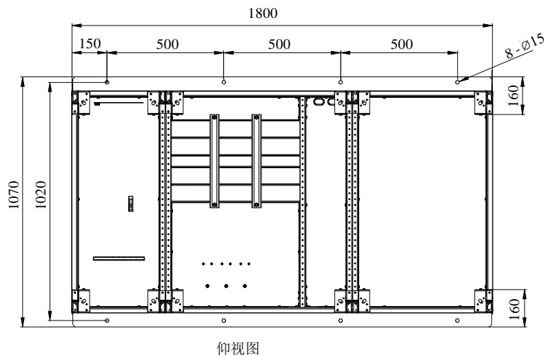
图2-9 带防震组件的安装示意图（底视图）
