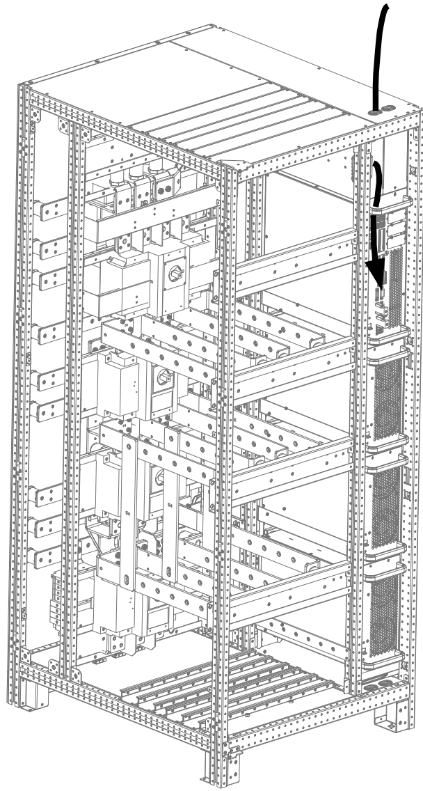
图3-11 600kVA 信号电缆进线示意图（上进线）
