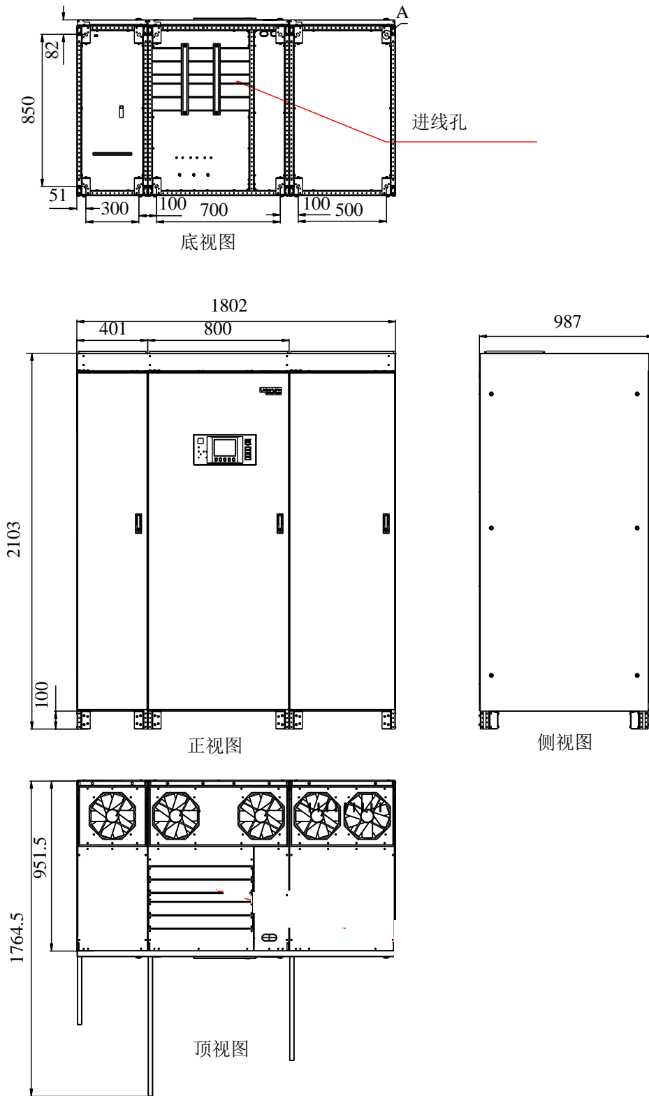
图8-9 600kVA 含上出风风扇的机柜安装尺寸示意图 (单位: mm)
