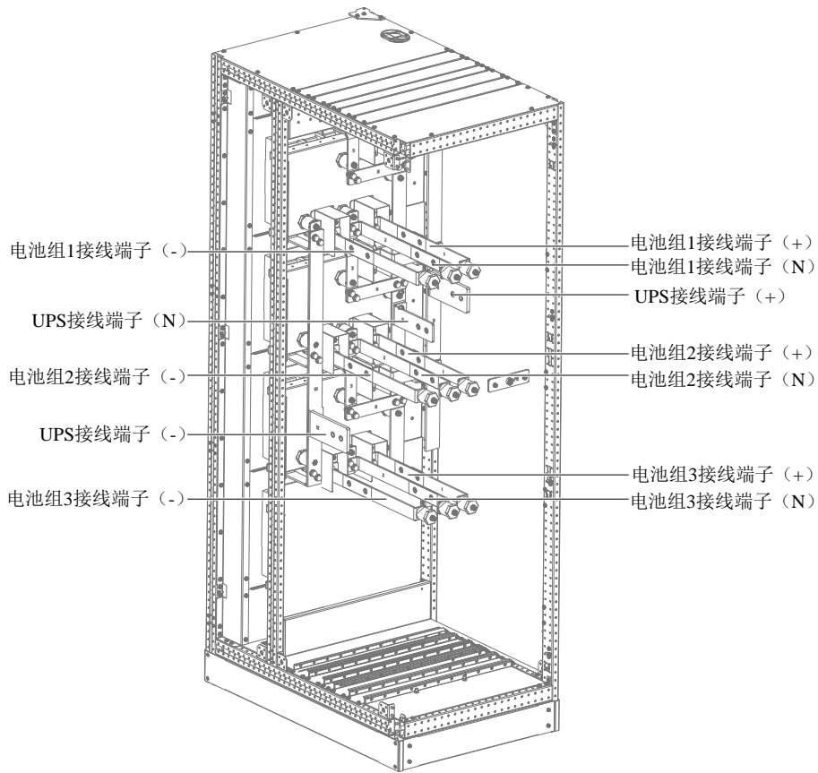
图6-6 分3组电池开关柜内部接线端子说明
