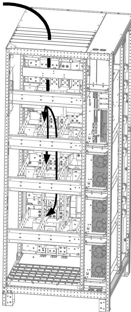
图3-3 600kVA 功率电缆走线示意图（上进线）
