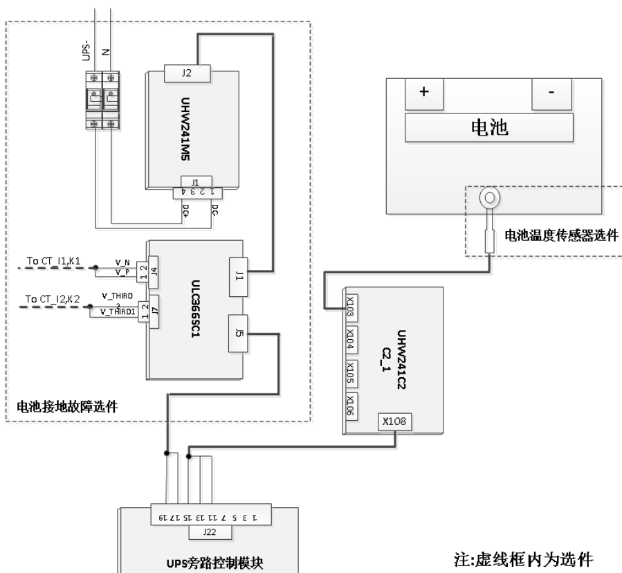
图6-8 总体 BCB 开关柜内部接线图及选件部分接线图
