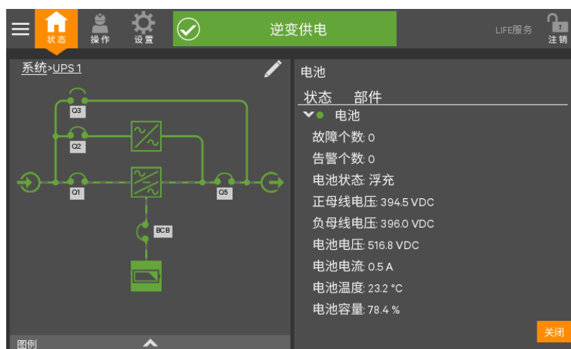
图4-39 本机状态--电池详情
