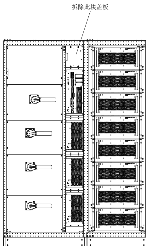
图8-7 拆盖板示意图
