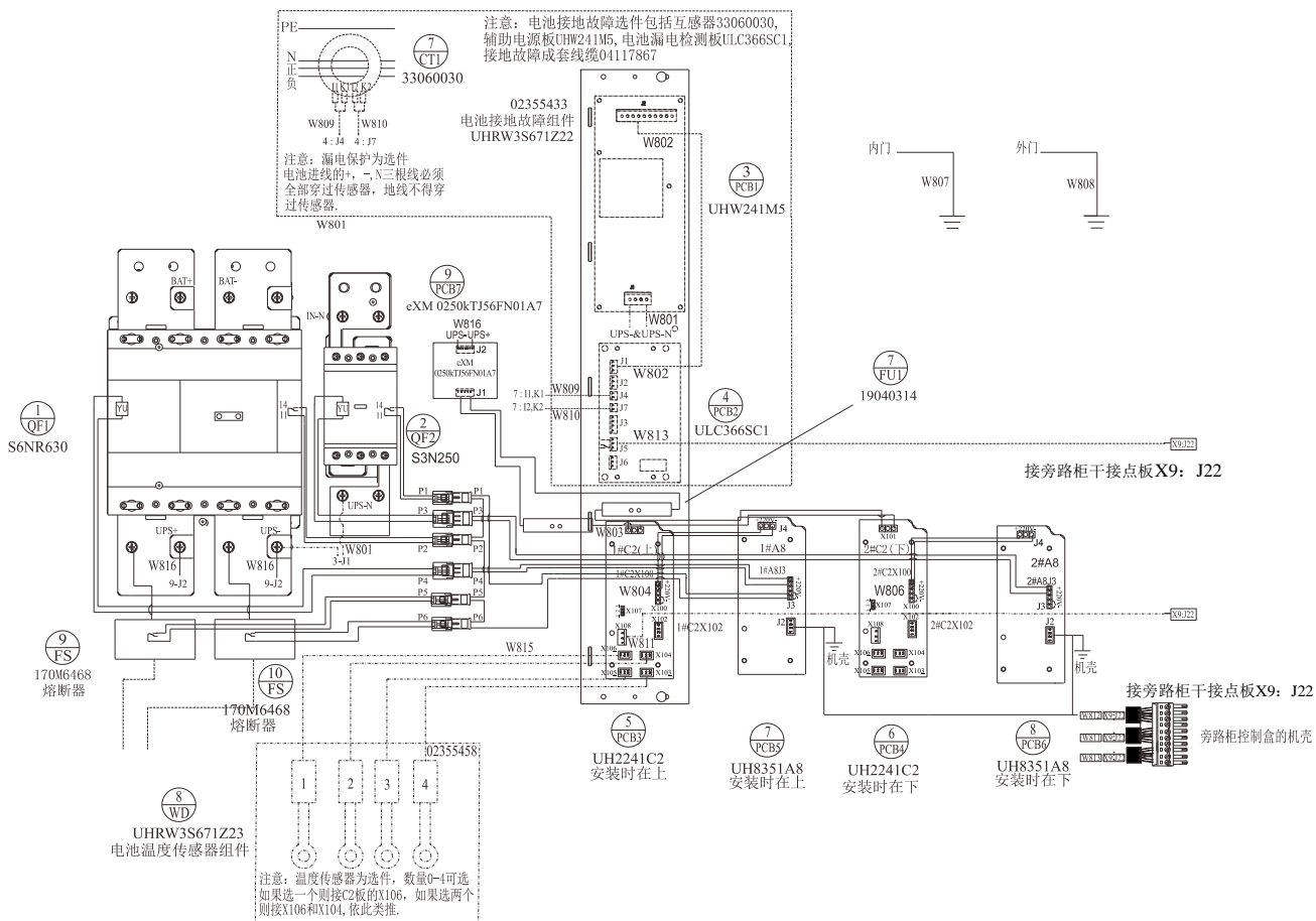
图6-5 电池开关盒接线图 BCB 参考电流与连接
