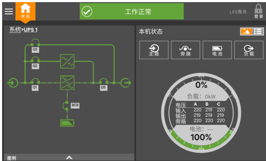
图4-2 开机后的主界面
