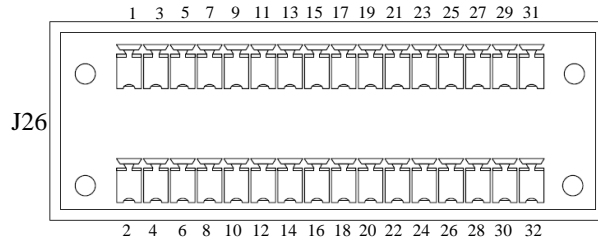
图3-8 干接点接口 J26 示意图
