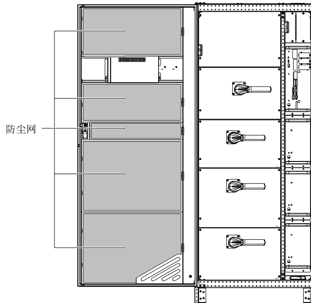
图10-1 更换防尘网
