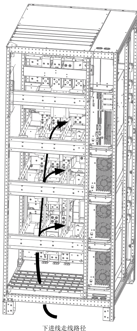
图3-4 400kVA 功率电缆走线示意图（下进线）
