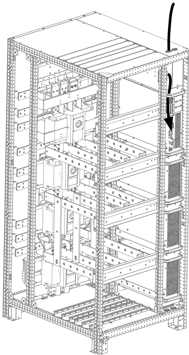
图3-11 400kVA 信号电缆进线示意图（上进线）
