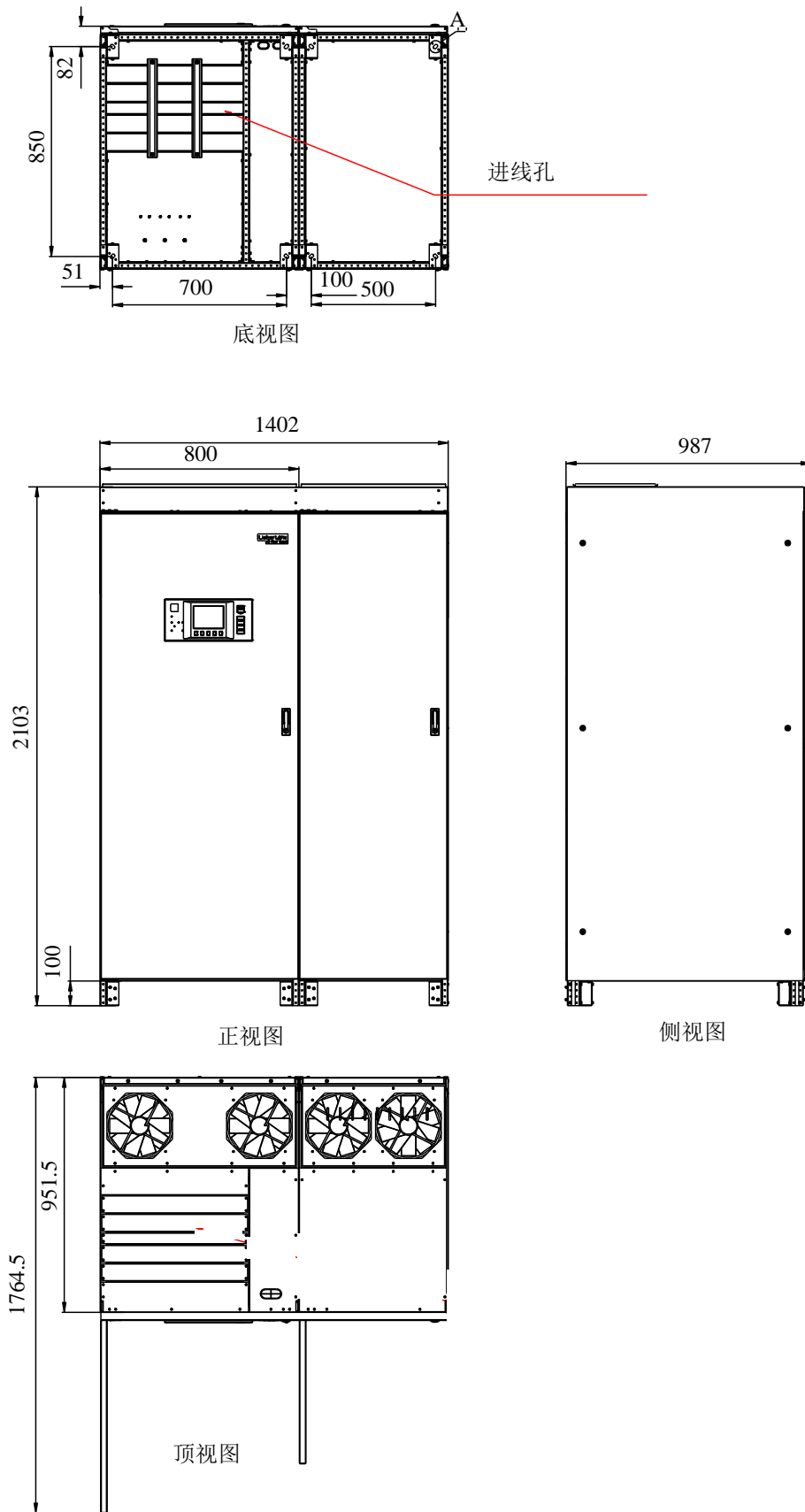
图8-8 400kVA 含上出风风扇安装尺寸图 (单位: mm)
