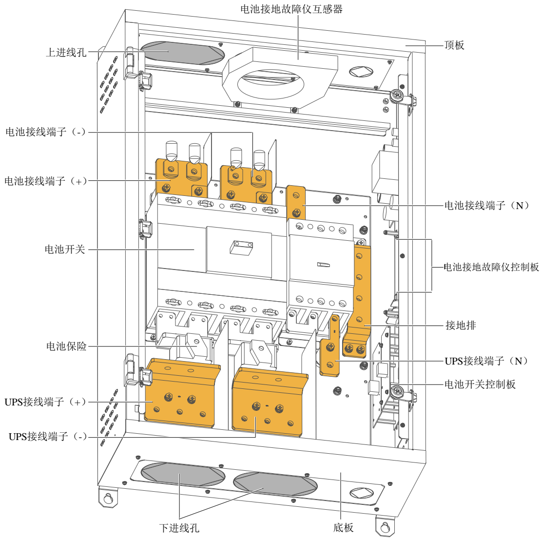
图6-4 电池开关盒内部结构
