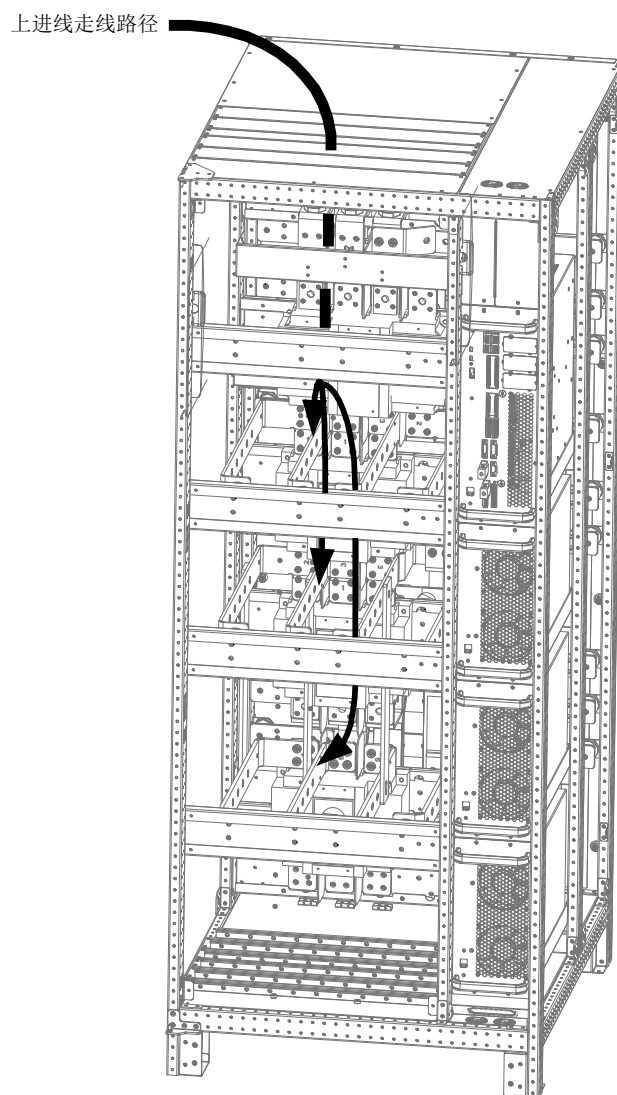
图3-3 400kVA 功率电缆走线示意图（上进线）
