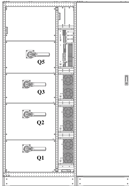
图5-1 UPS 电源开关位置示意图
