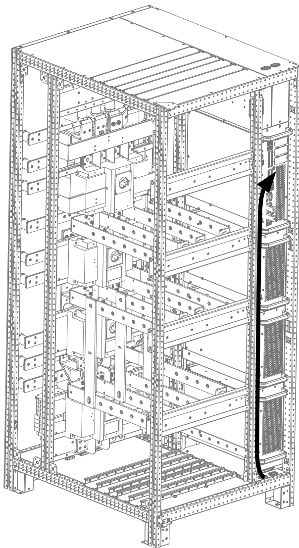
图3-12 400kVA 信号电缆进线示意图（下进线）
