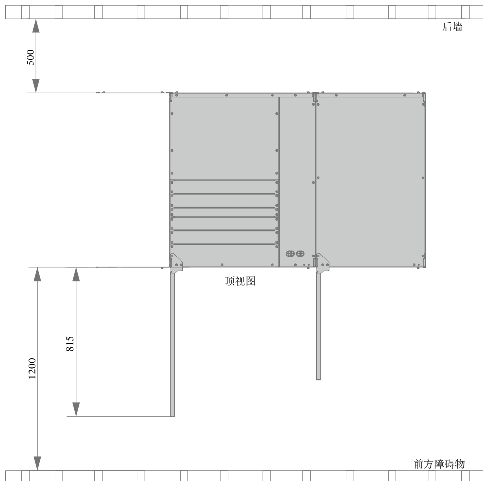
图2-6 操作空间示意图（单位：mm）
