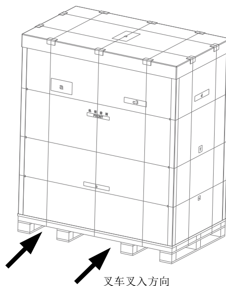
图2-1 叉车叉入示意图（机柜前部）
