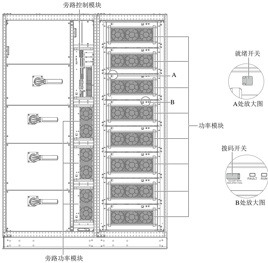
图2-7 400kVA 功率模块安装示意图
