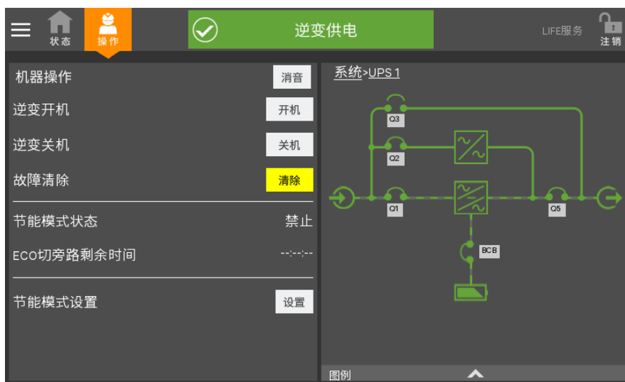
图5-5 完成开机
