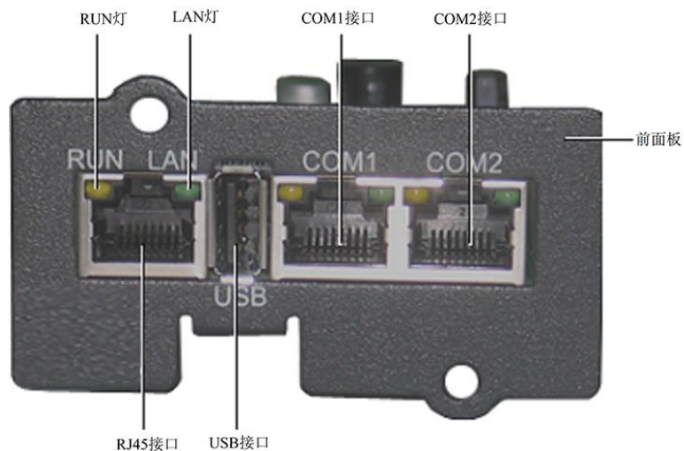
图8-4 SIC卡外观
