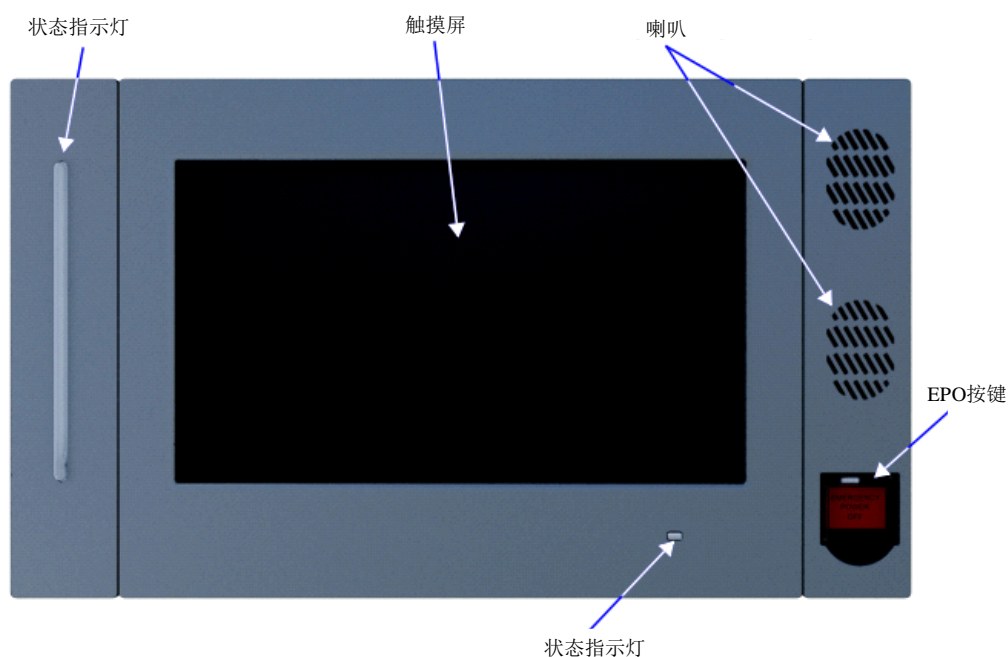
图4-1 触摸屏外观
