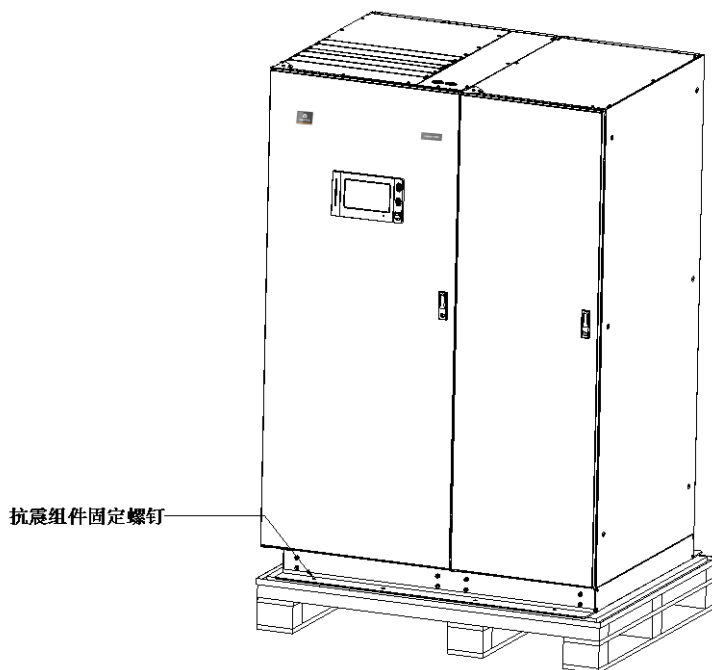
图2-5 拆除防震组件固定螺栓（前后共 8 个）
