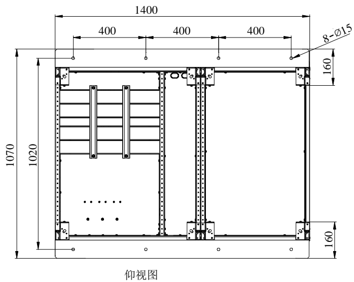
图2-9 带防震组件的安装示意图（底视图）
