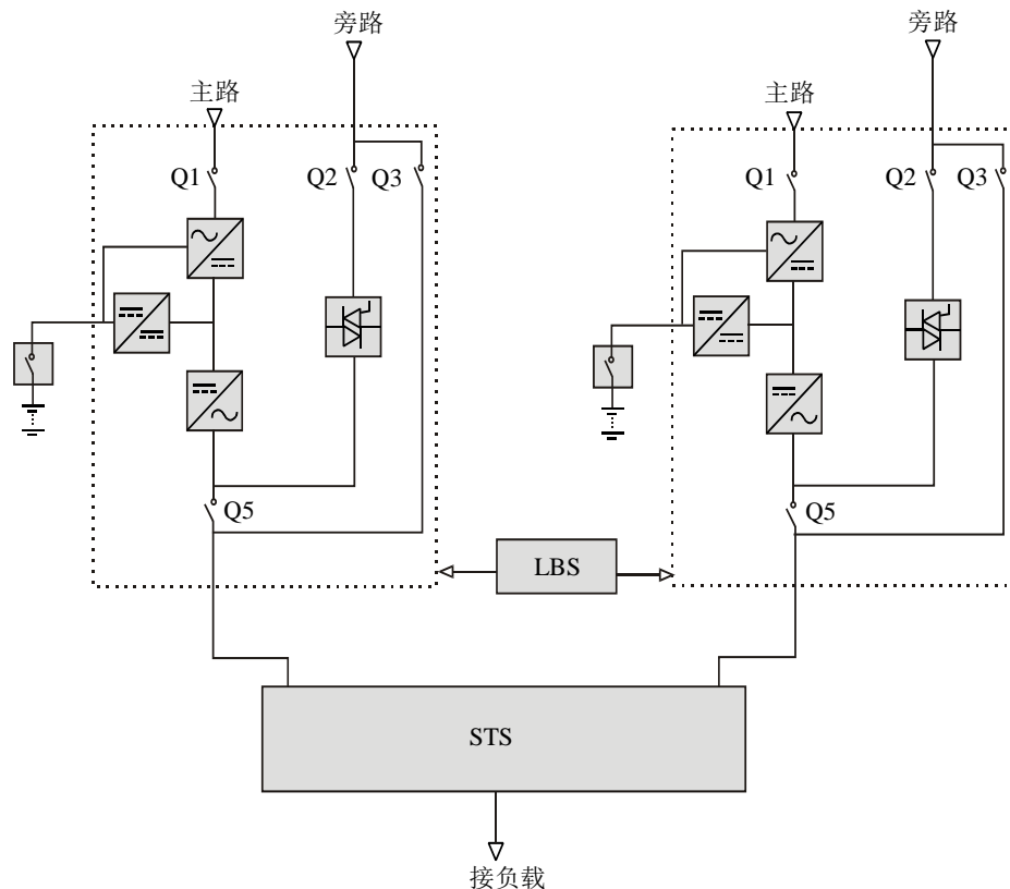
图 7-7 典型双母线系统
