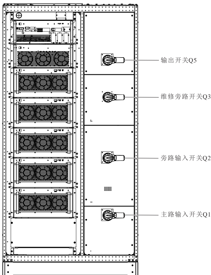
图5-1 UPS 电源开关位置示意图
