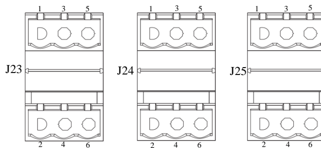
图3-9 干接点接口 J23~J25 示意图
