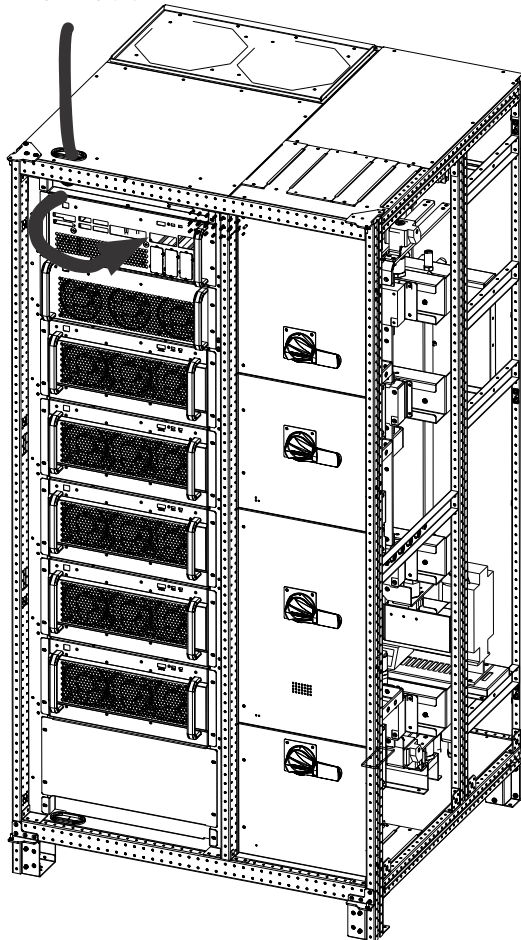
图3-11 信号电缆走线示意图（上进线）
