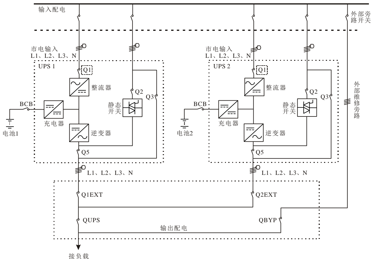
注：主路输入开关Q1、旁路输入开关Q2、输出开关Q5为选配，维修旁路开关Q3为标配。
