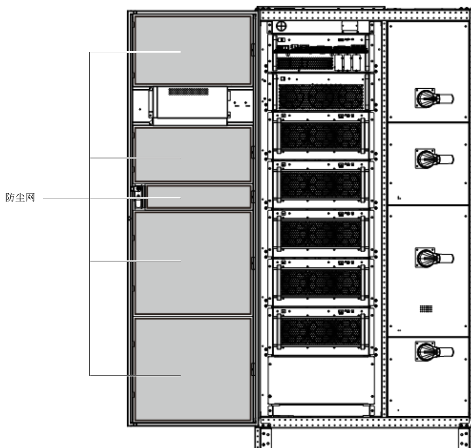
图10-1 更换防尘网
