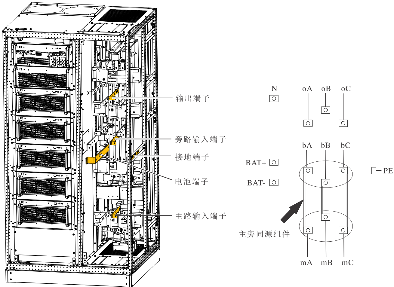
图3-2 250kVA UPS 功率电缆接线端子示意图
