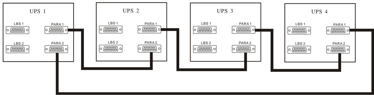
图7-2 并机系统并机电缆连接
