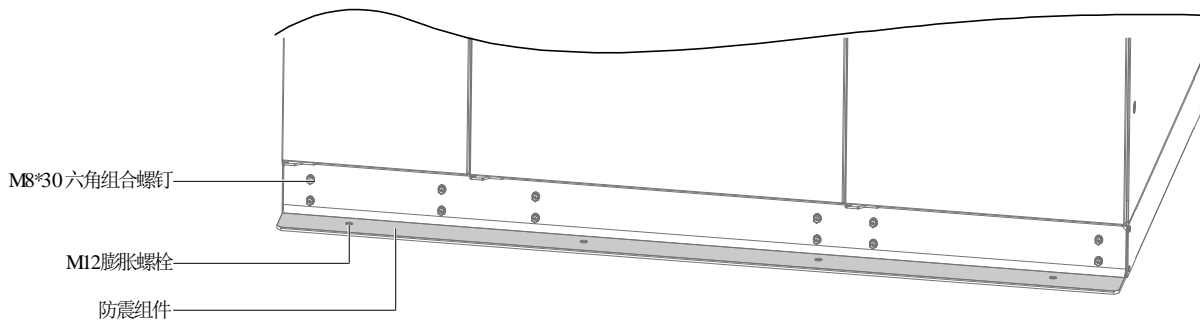
图8-1 防震选件安装示意图
