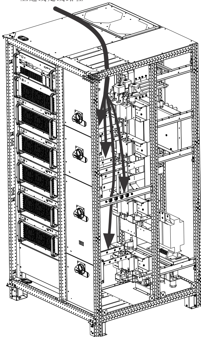
图3-3 功率电缆走线示意图（上进线）
