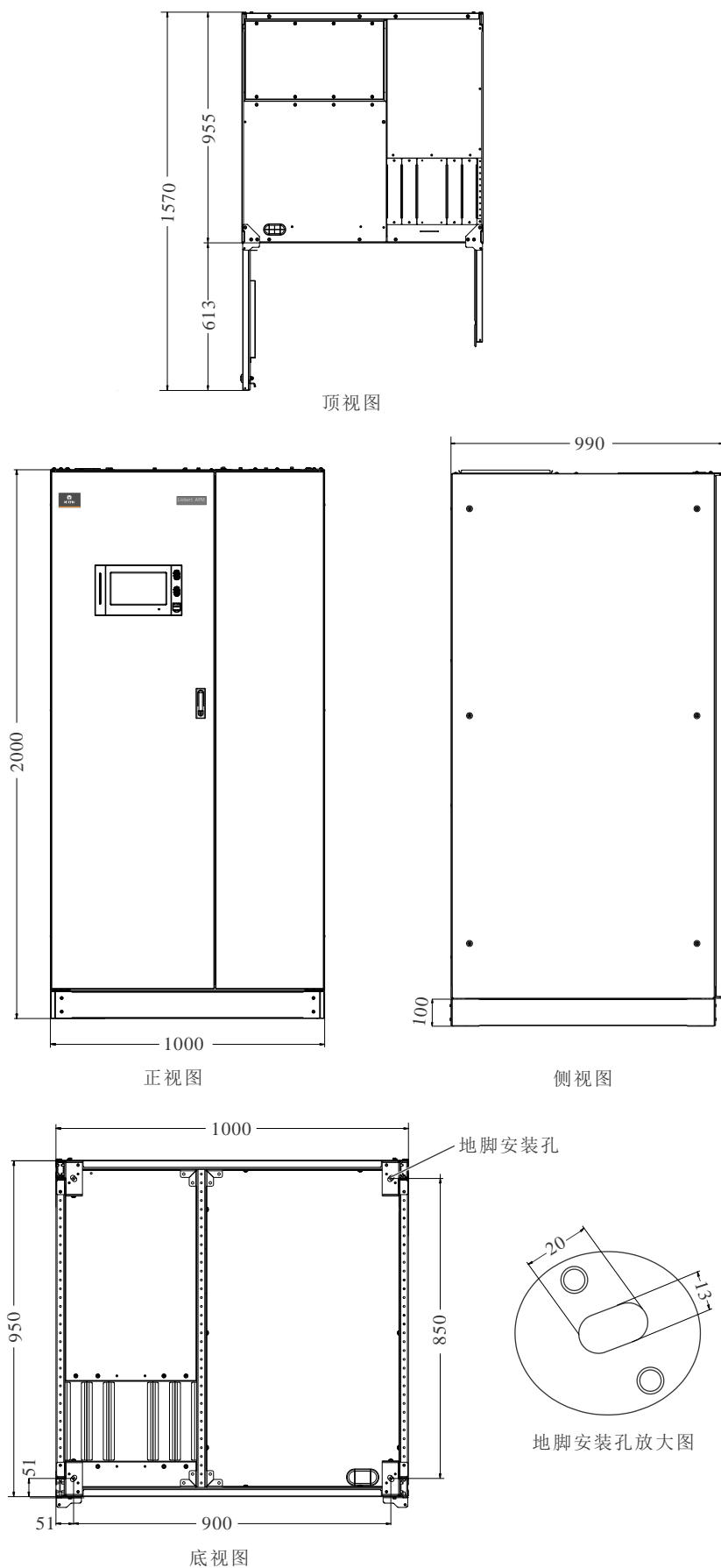
图2-8 250kVA 安装尺寸示意图 (单位: mm)
