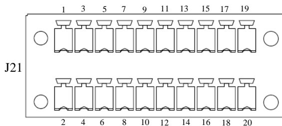
图3-6 干接点接口 J21 示意图
