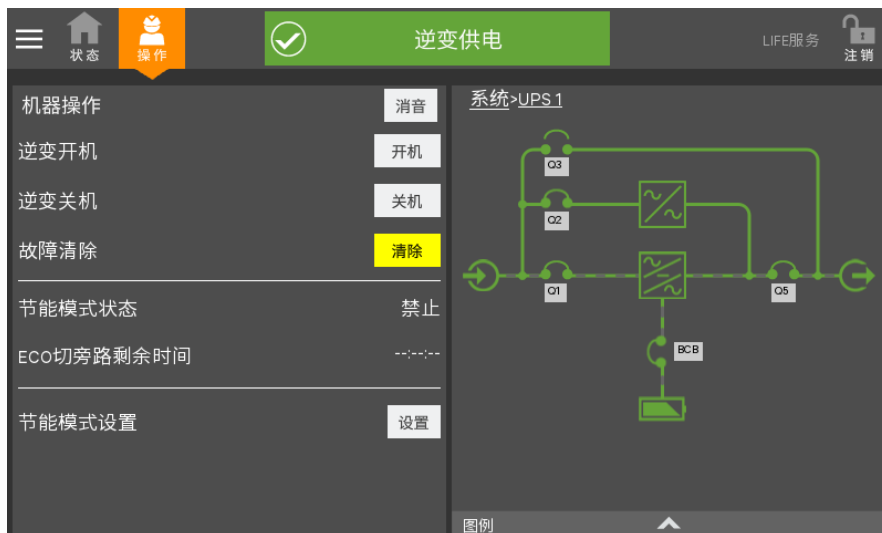
图5-5 完成开机
