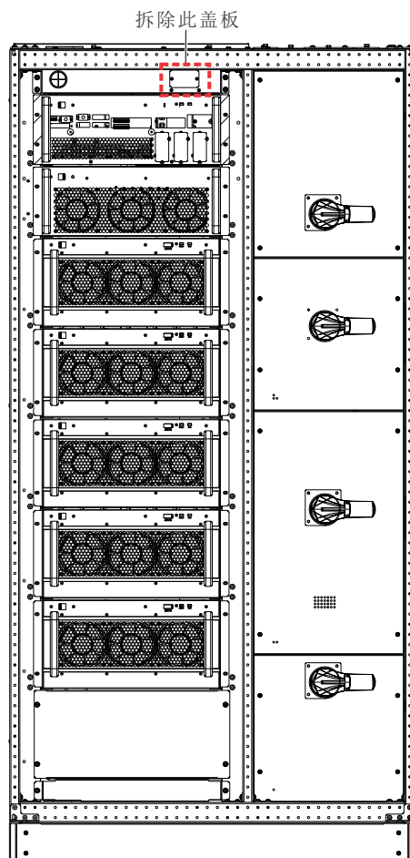
图8-7 拆盖板示意图
