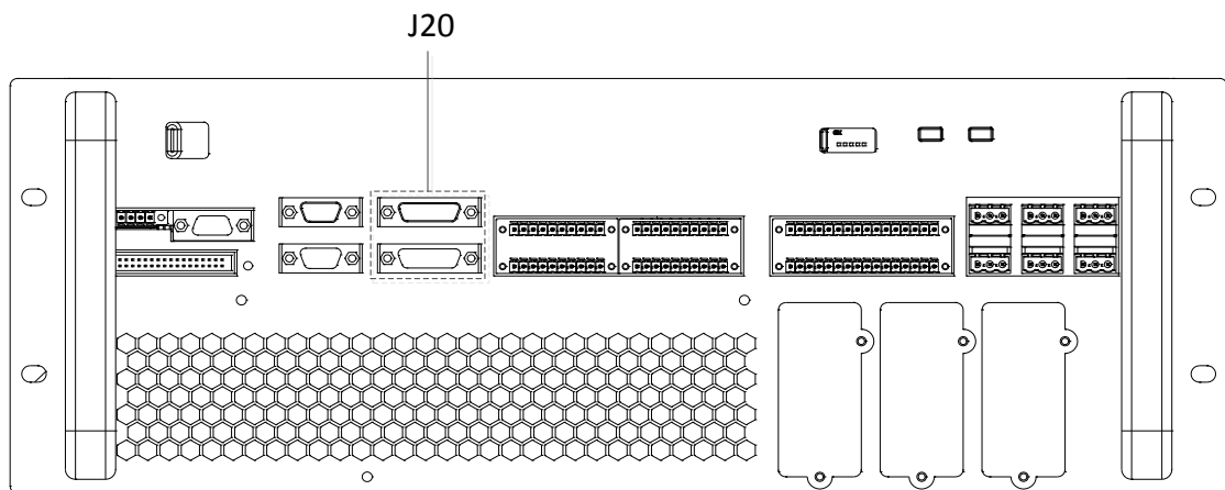
图7-3 旁路控制模块并机接口（J20）图
