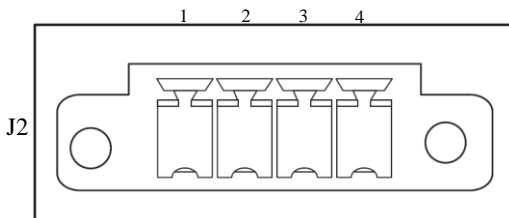
图3-10 REPO 接口 J2 示意图
