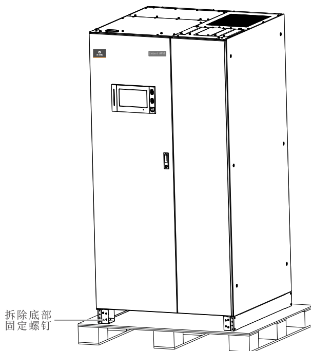
图2-4 拆除机柜地脚螺栓
