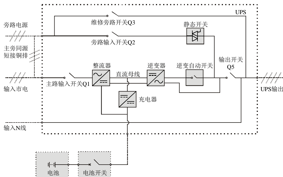
图 1-2 UPS 电源开关配置
