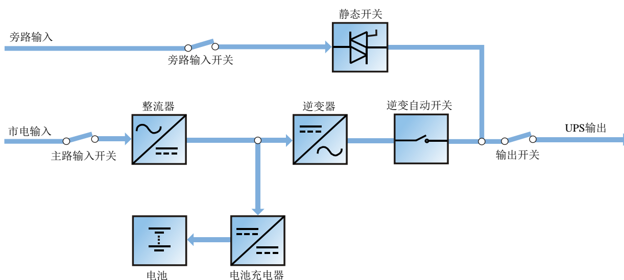
图1-7 ECO 模式
