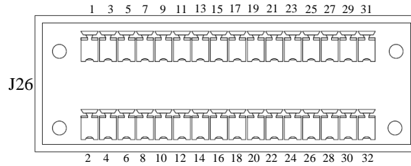
图3-8 干接点接口 J26 示意图
