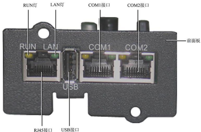
图8-4 SIC卡外观
