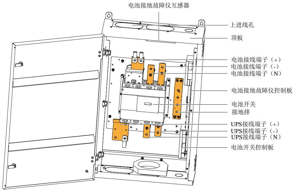
图6-4 电池开关盒内部结构
