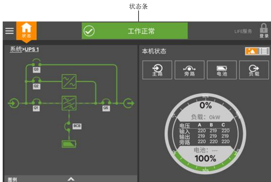
图4-40 状态条
