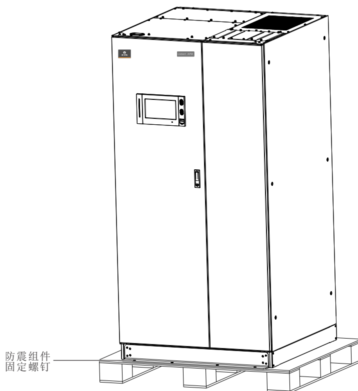
图2-5 拆除防震组件固定螺栓（前后共 8 个）
