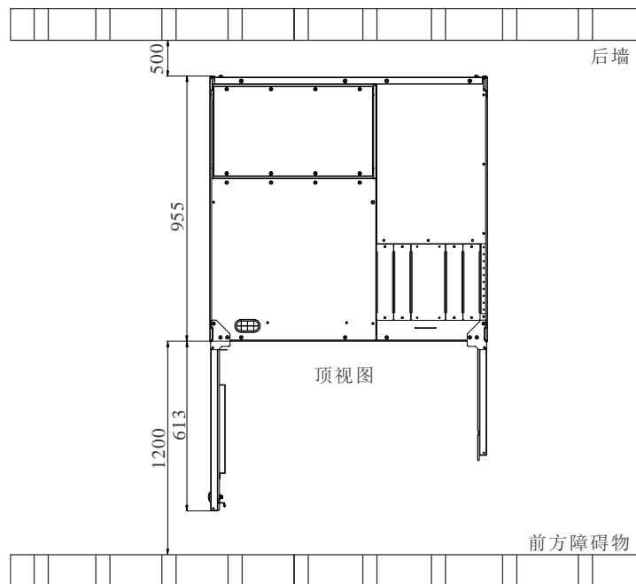
图2-6 操作空间示意图 (单位: mm)
