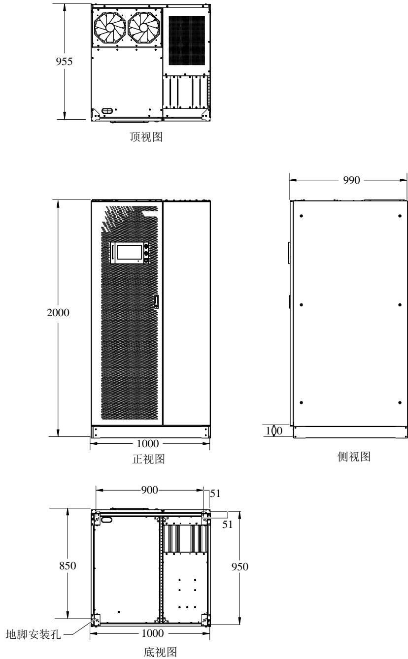
图8-8 250kVA 含上出风风扇安装尺寸图 (单位: mm)
