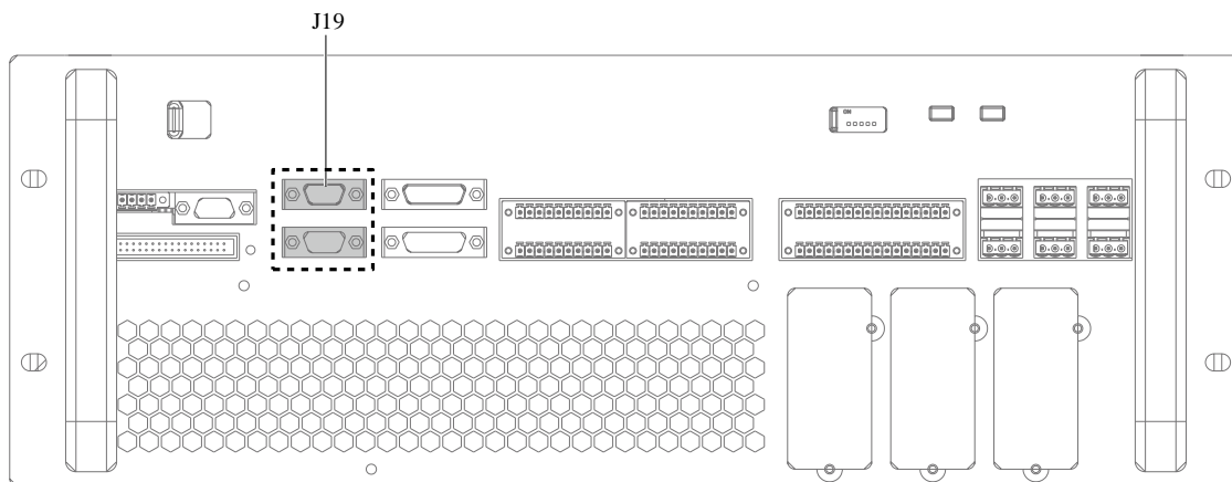
图7-9 旁路控制模块 LBS 接口（J19）图
