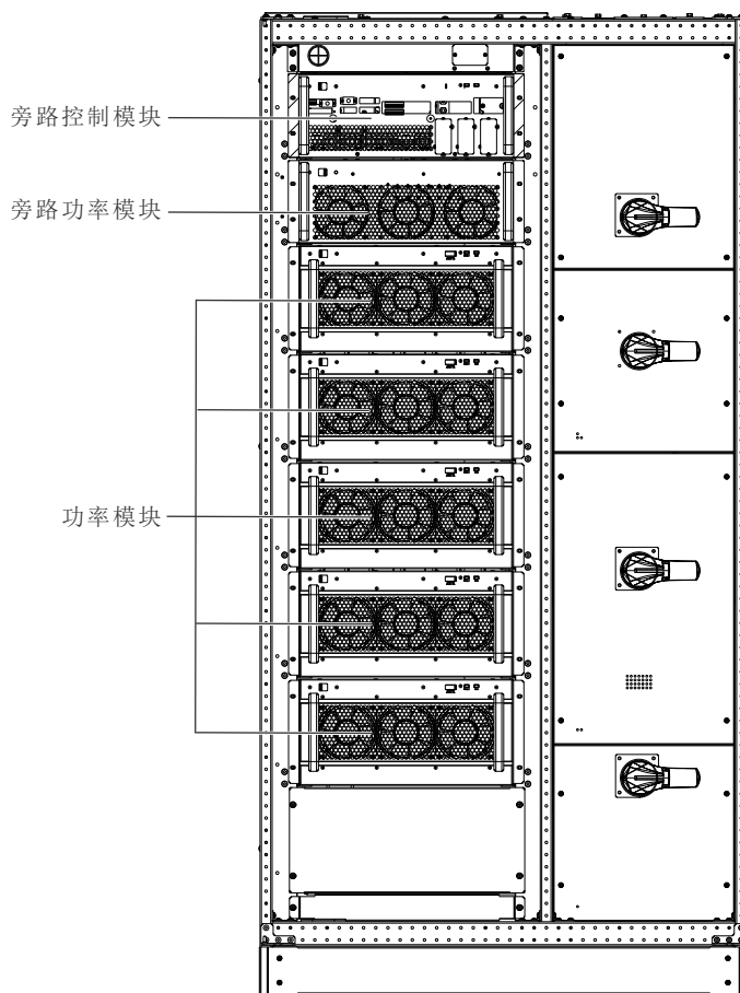
图2-7 250kVA 功率模块安装示意图
