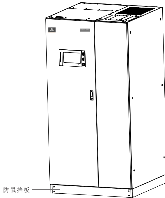
图2-3 拆除防鼠板
