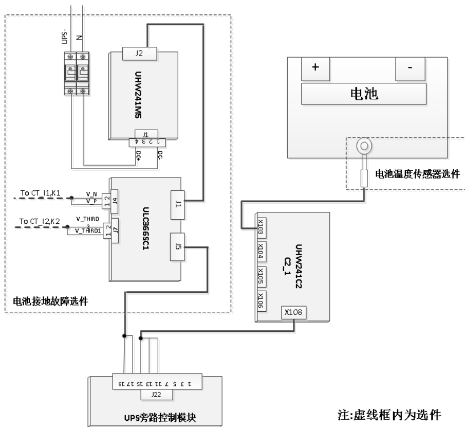
图6-5 总体 BCB 开关柜内部选件接线图
