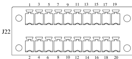
图3-7 干接点接口 J22 示意图
