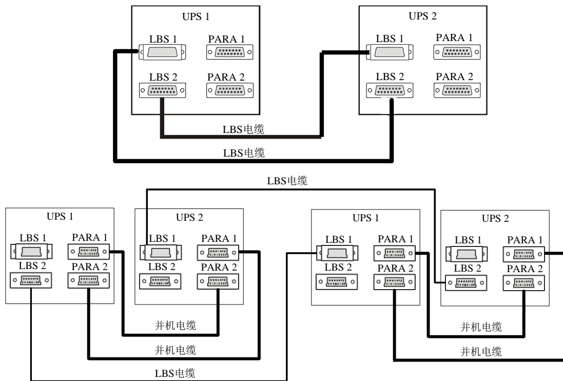
图7-8 典型双母线系统的 LBS 电缆连接（单机、并机）
