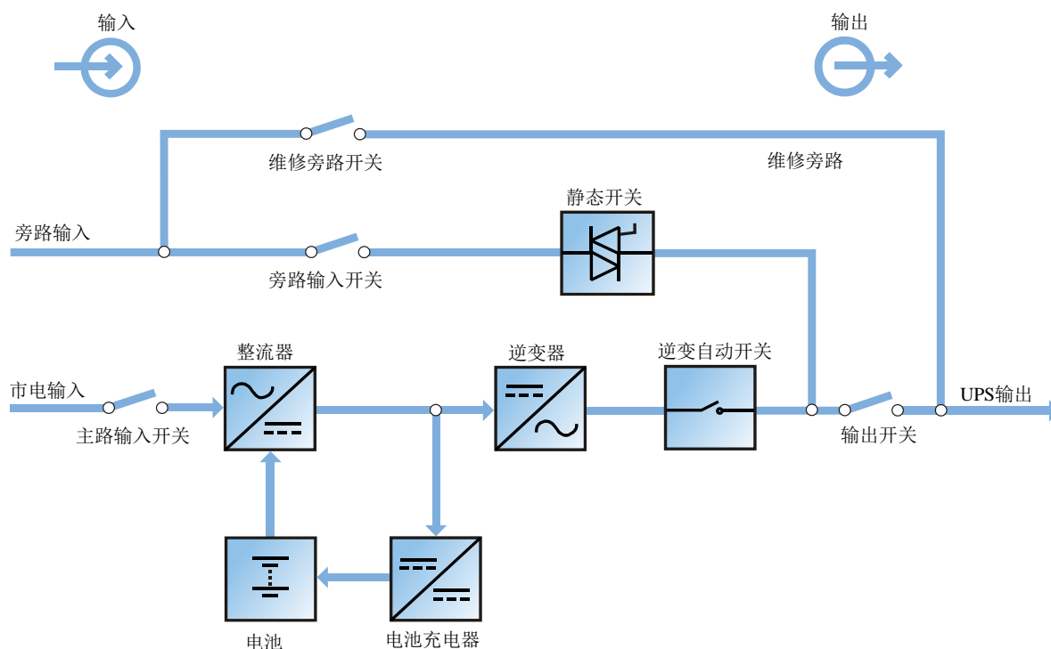
图1-1 UPS 单机工作原理框图
