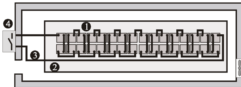
图6-2 电池房设计
