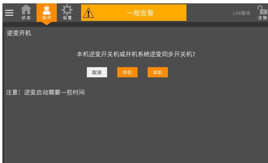
图7-5 并机系统 UPS 同步开机
