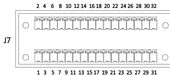
图 3-6 干接点接口 J7 示意图
