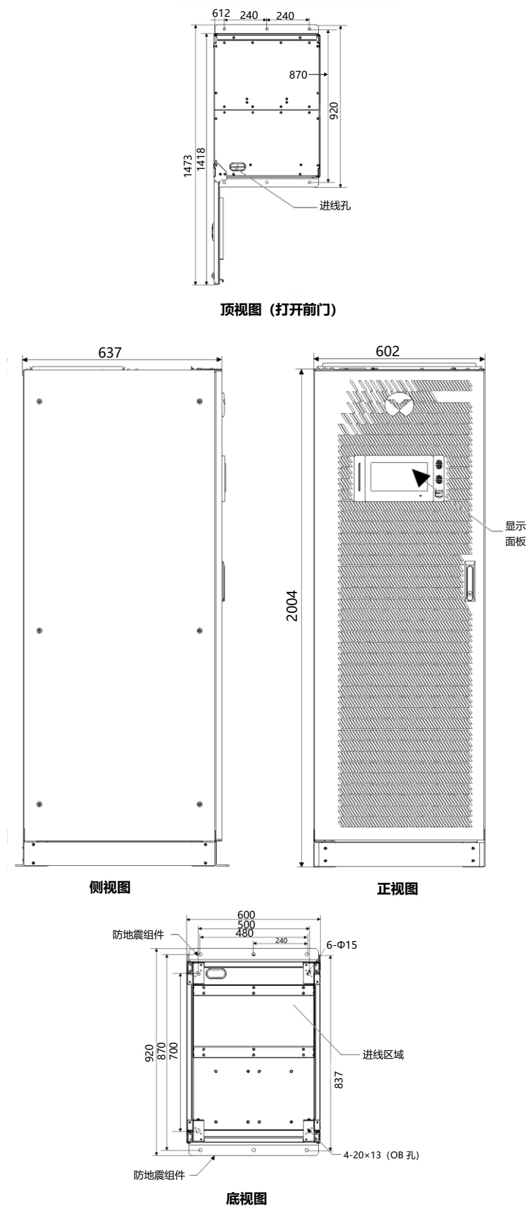
图2-7 250kVA 安装尺寸示意图 (单位: mm)
