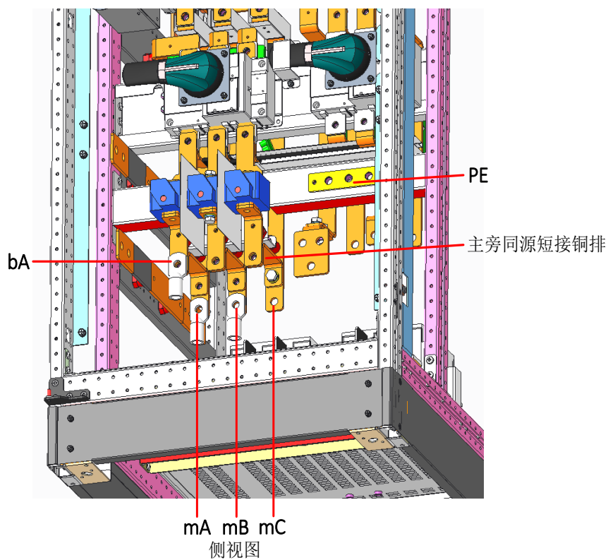
250kVA 接线端子示意图
