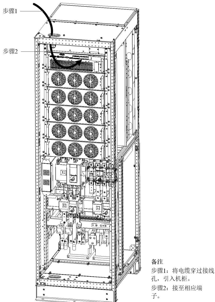
图3-9 250kVA 信号电缆走线示意图 (上进线)
