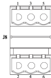
图3-7 干接点接口 J8 示意图
