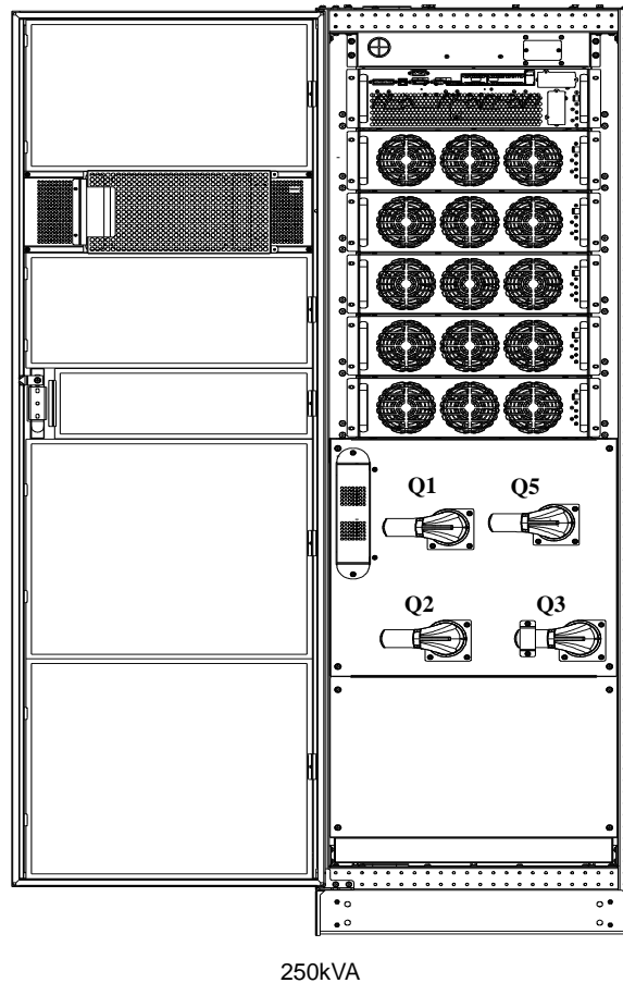
图5-1 UPS 电源开关位置示意图
