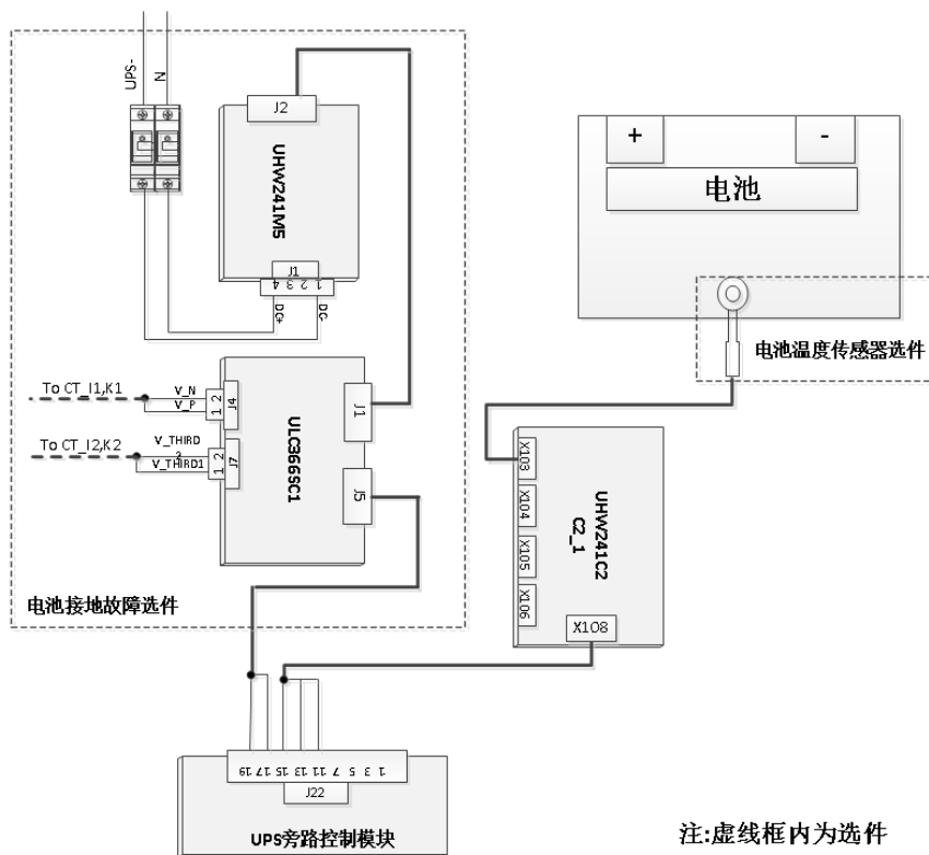
图 6-5 总体 BCB 开关柜内部选件接线图
