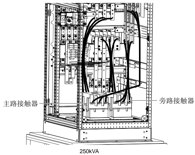
图8-5 反灌接触器接线示意图
