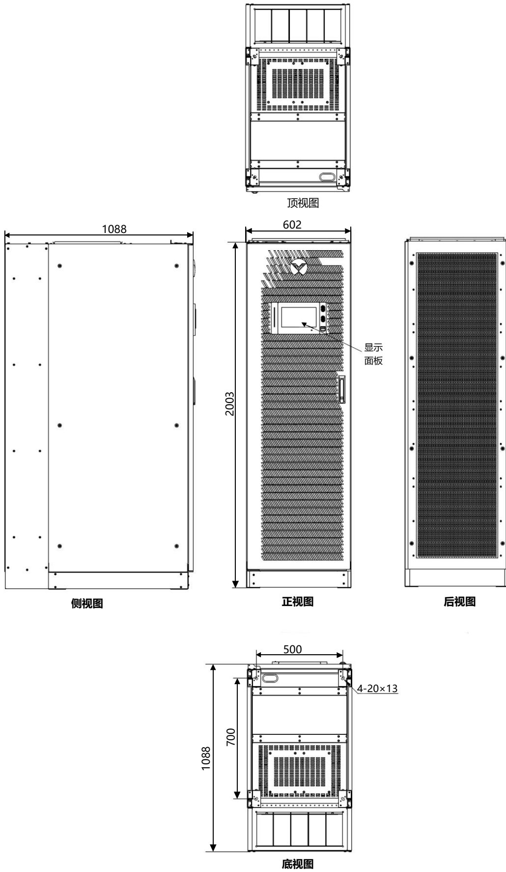
图2-8 250kVA 加深机柜安装尺寸示意图 (单位: mm)
