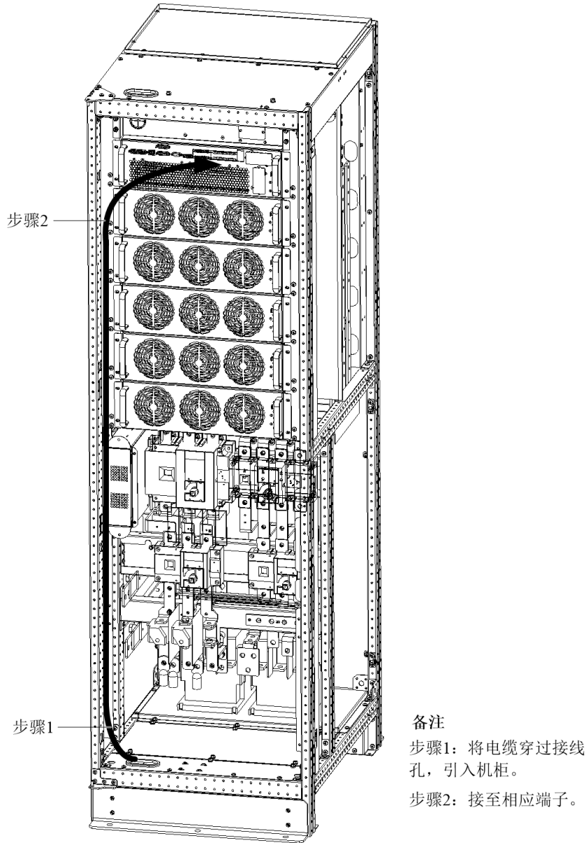
图3-10 250kVA 信号电缆走线示意图（下进线）
