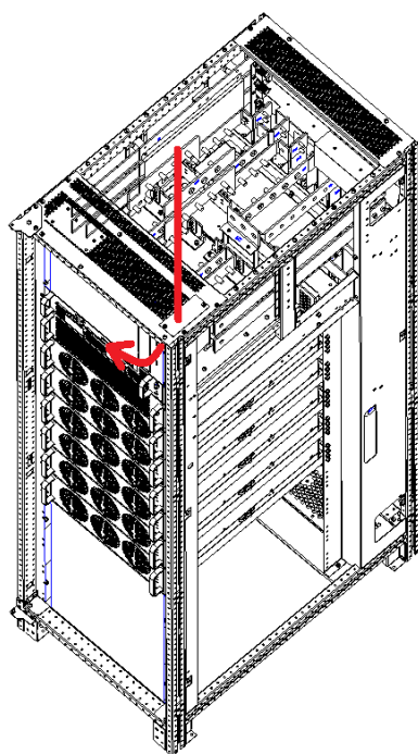
图 3-9 无开关信号电缆走线示意图
