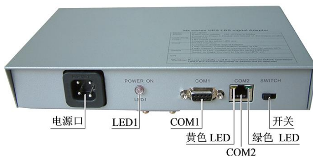
图 8-7 IS-RELAY 卡外观图
