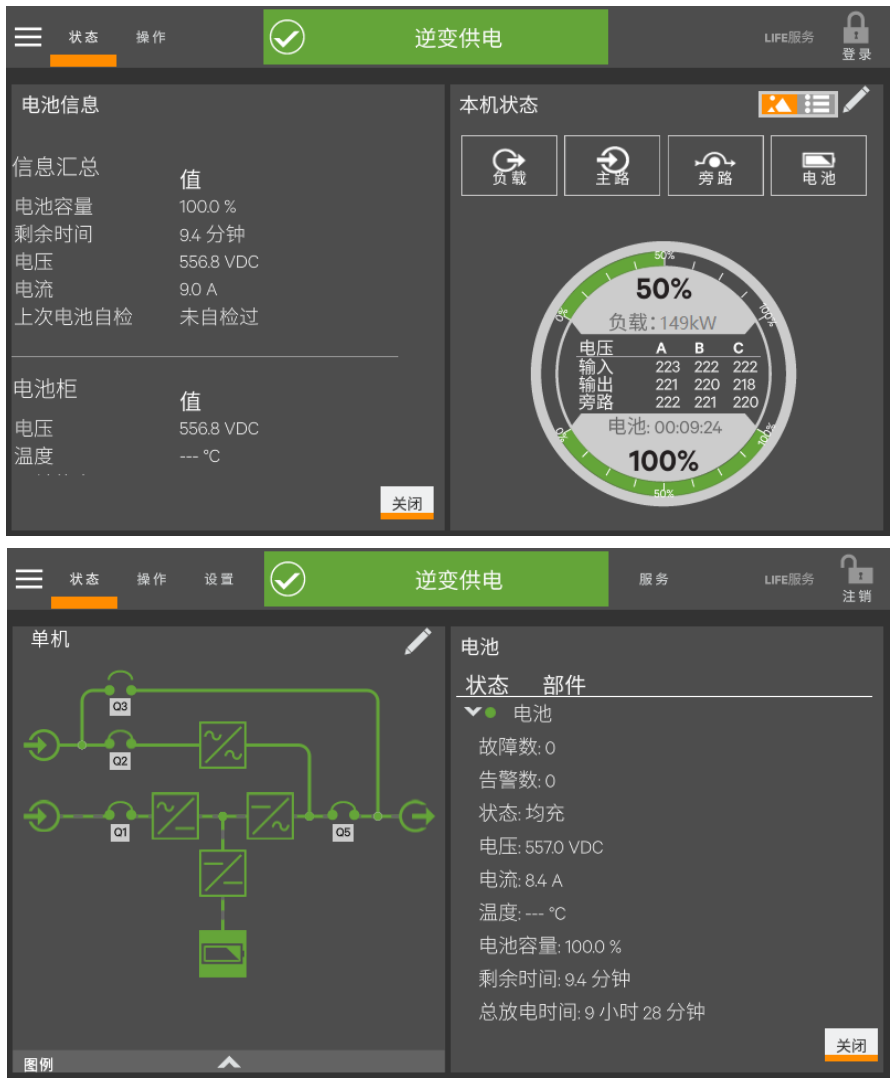
图 4-30 本机状态--电池详情
