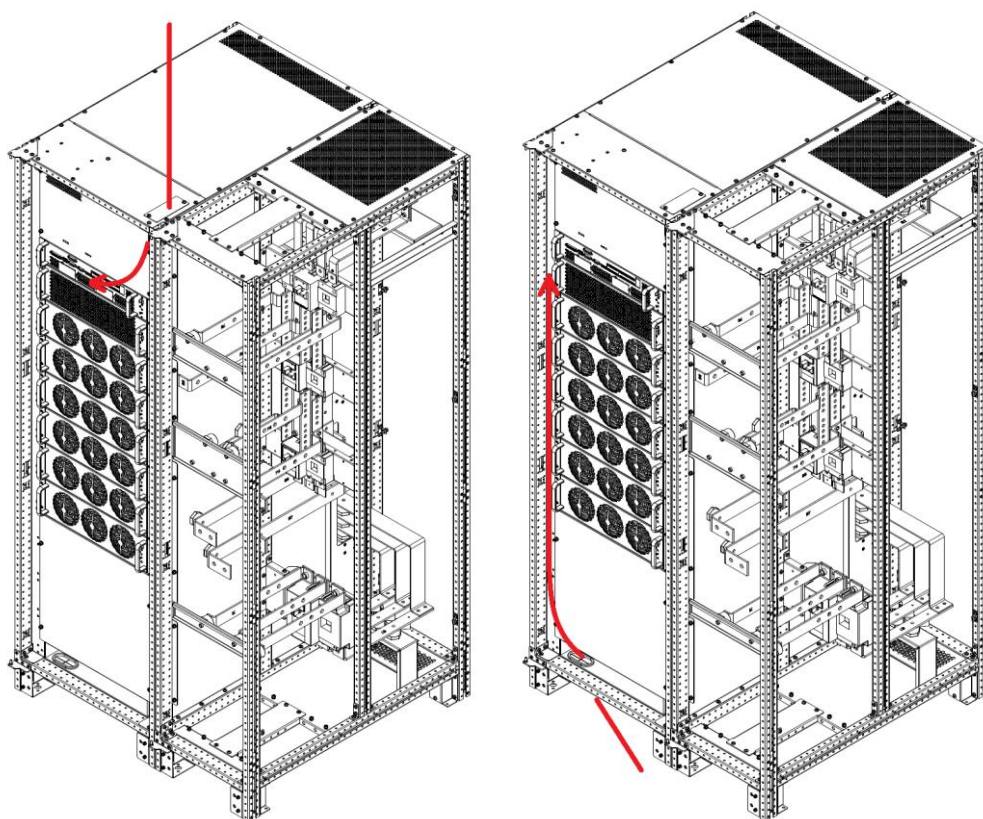
图 3-10 四开关信号电缆走线示意图（上进线、下进线）
