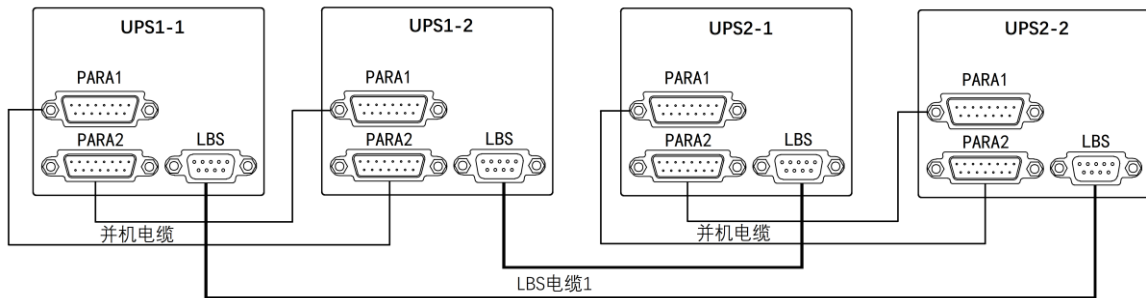
图 7-9 典型同步双母线系统的 LBS 电缆连接 (并机)
