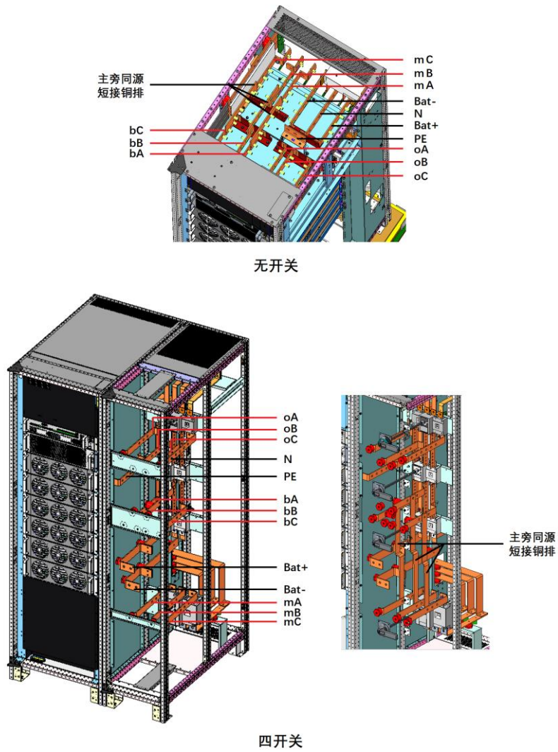
图 3-2 UPS 机柜功率电缆连接端子示意图
