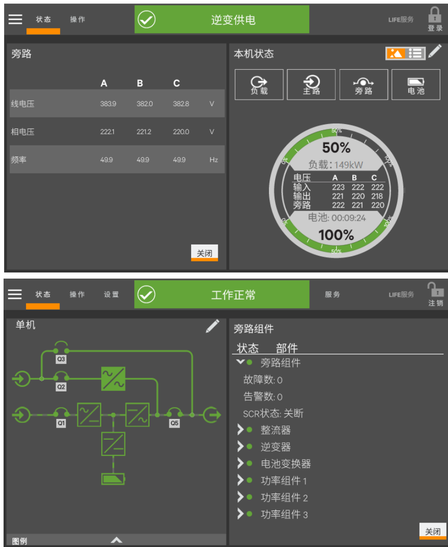
图 4-29 本机状态--旁路详情
