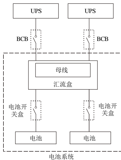
图 6-2 公用电池组接线示意图
