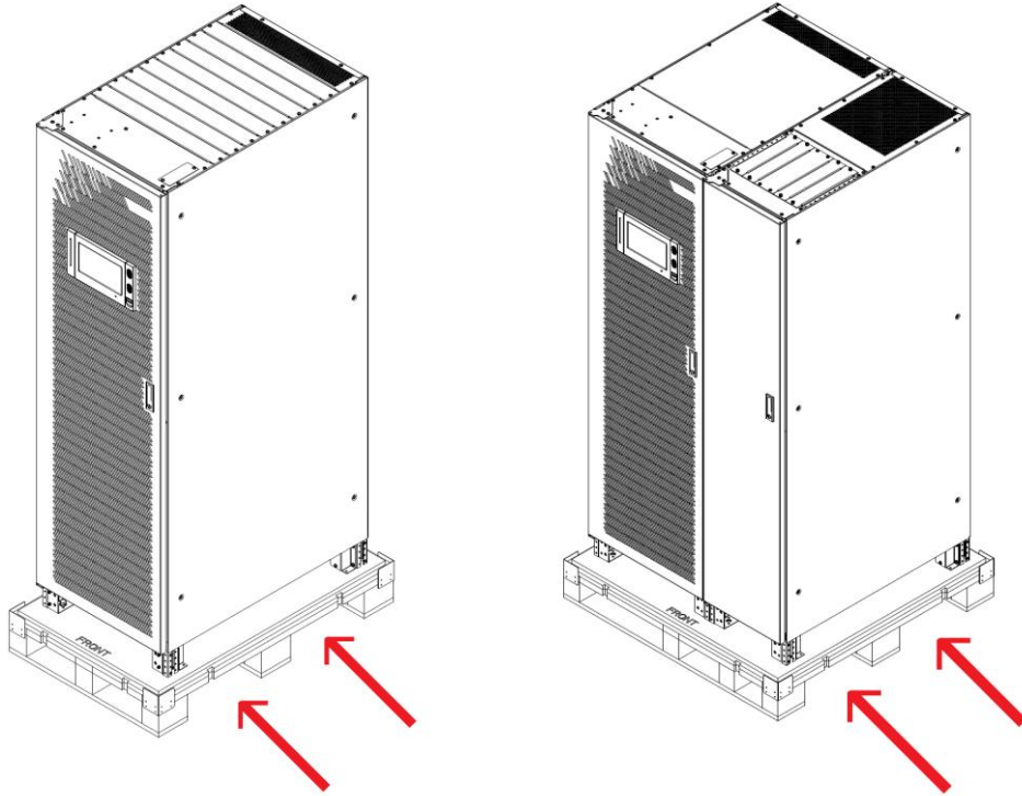
图 2-1 叉车叉入方向及运输示意图
