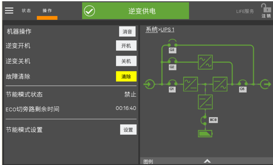
图 5-9 切换 UPS 至正常模式
