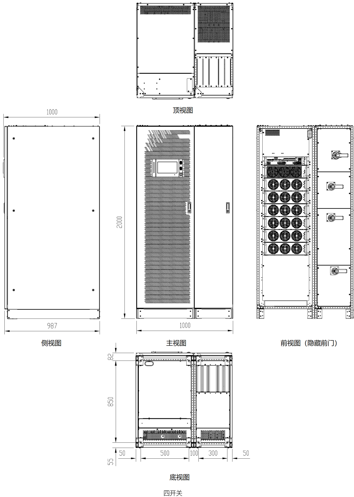
图 2-5 300kVA 无开关、四开关安装尺寸示意图 (单位: mm)
