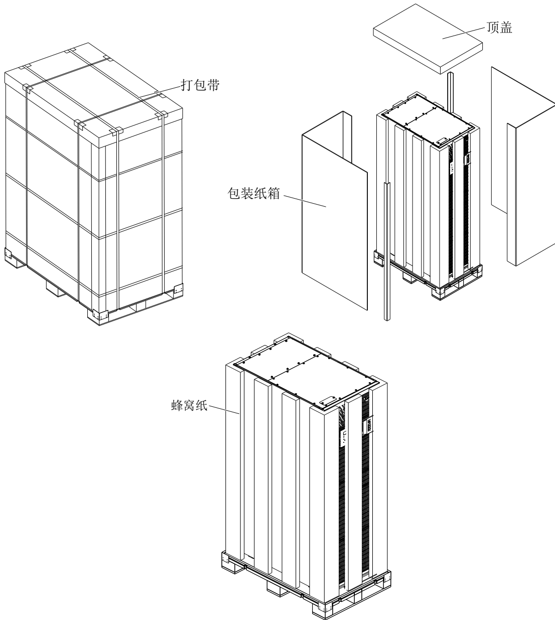
图 2-2 拆除打包带及纸顶盖和包装纸箱，拆掉蜂窝纸板
