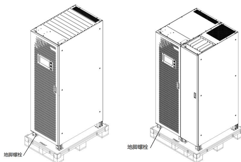
图 2-4 拆除机柜地脚螺栓
