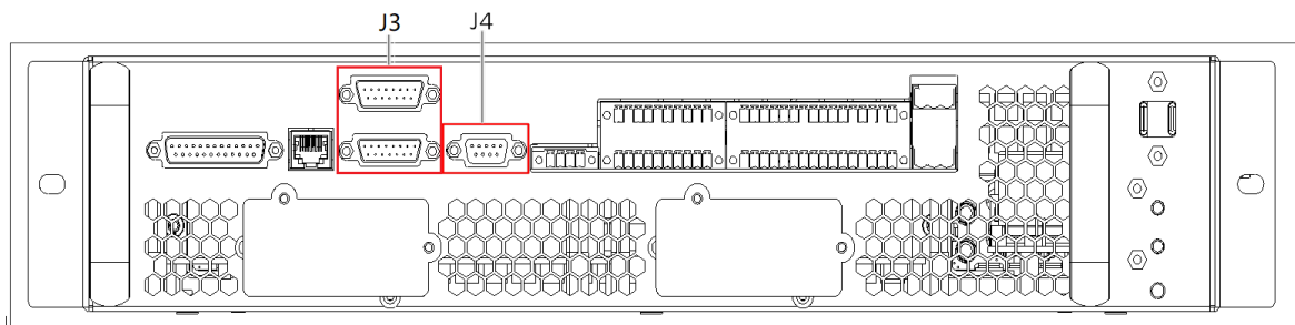
图 7-10 旁路模块 LBS 接口 (J4) 和 PARA 接口 (J3) 图
