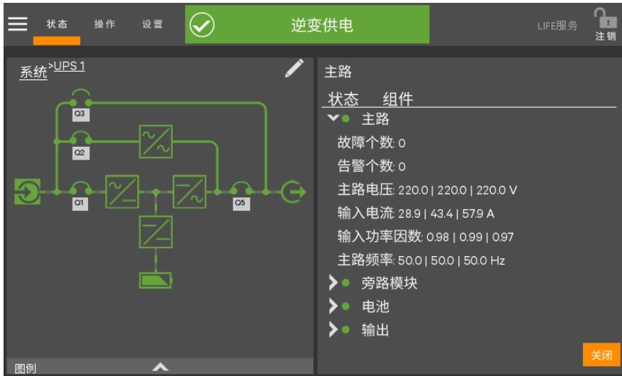
图 4-34 本机状态--输入详情
