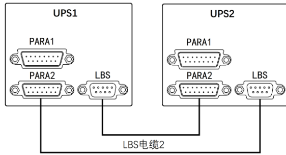
图 7-7 典型同步双母线系统的 LBS 电缆连接 (单机)
