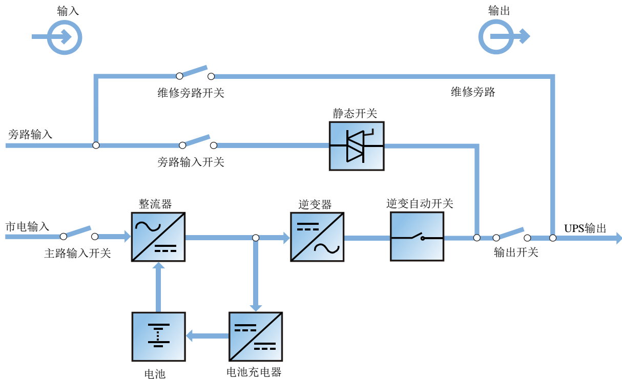
图1-1 UPS 单机工作原理框图 (无开关、四开关)
