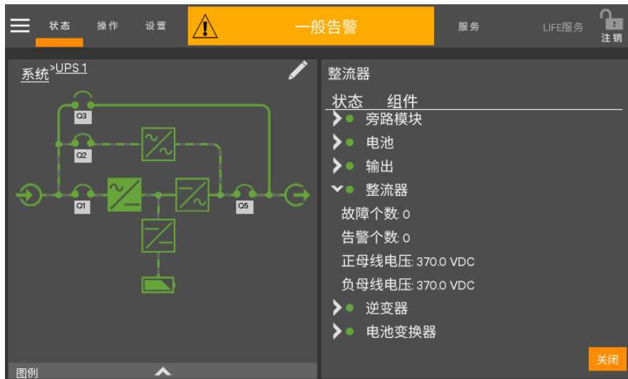
图 4-37 本机状态--整流器详情
