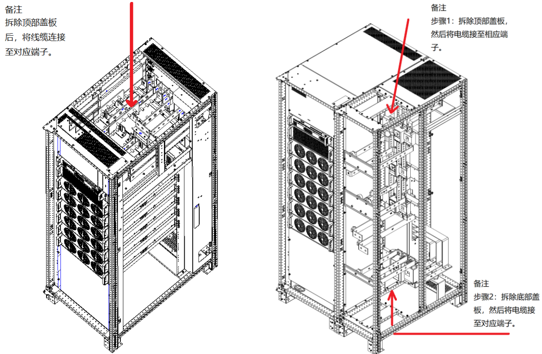
图 3-3 300kVA 功率电缆走线示意图
