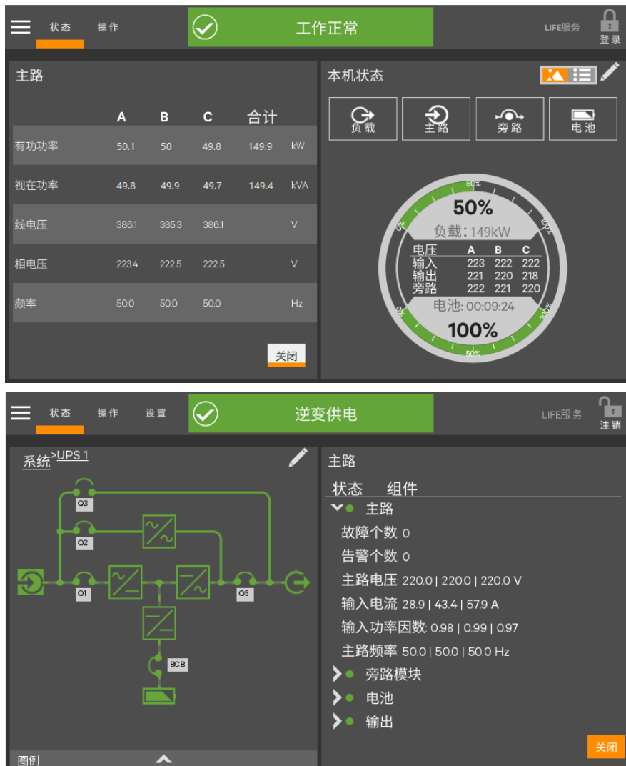
图 4-28 本机状态--输入详情
