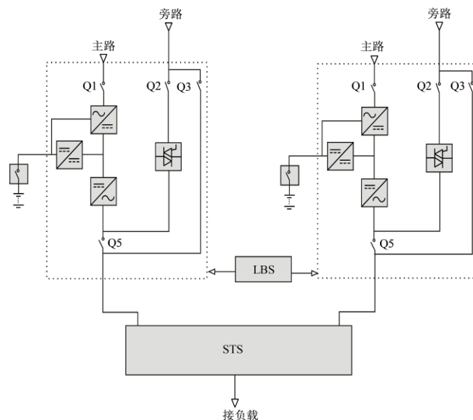
图 7-5 单机组成的典型双母线系统
