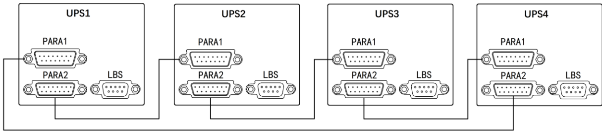
图 7-2 并机系统并机电缆连接
