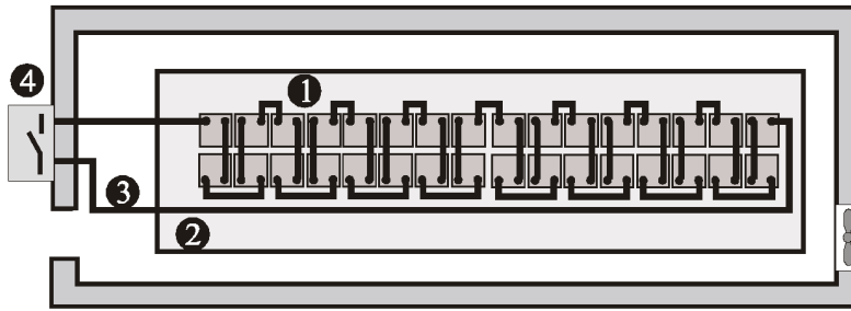
图 6-1 电池房设计
