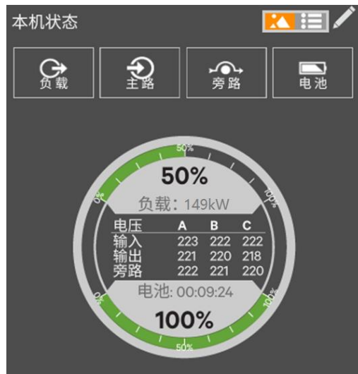
图 4-7 本机状态仪表盘
