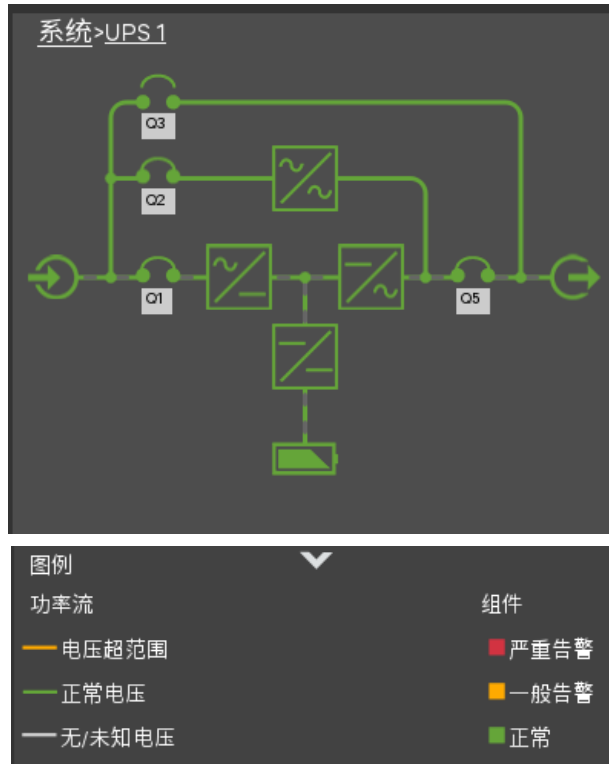
图 4-6 模拟显示，正常模式运行
