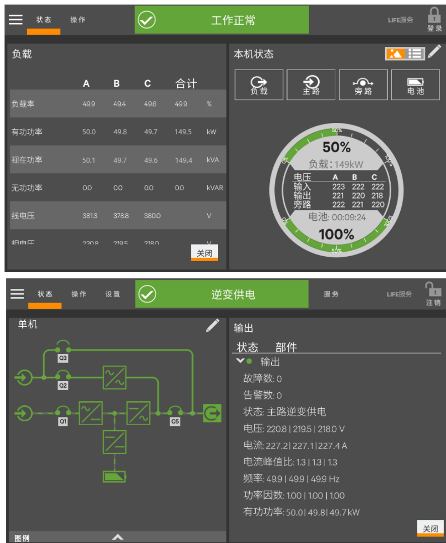
图 4-31 本机状态--负载详情
