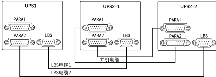
图 7-8 典型双母线系统的 LBS 电缆连接 (单机与并机)
