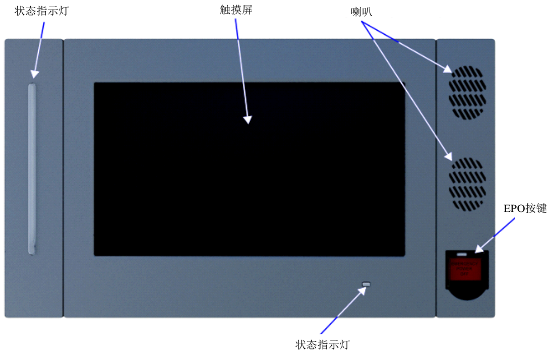
图 4-1 触摸屏外观
