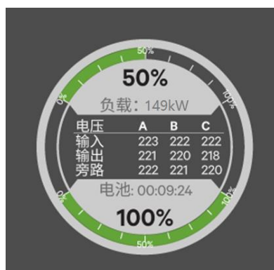
图 4-25 默认状态表视图
