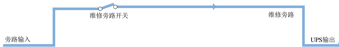
图 1-6 维修模式运行示意图
