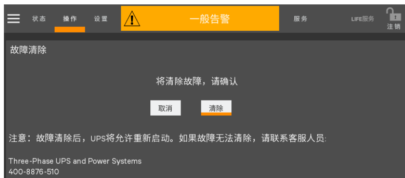
图 4-15 故障清除命令
