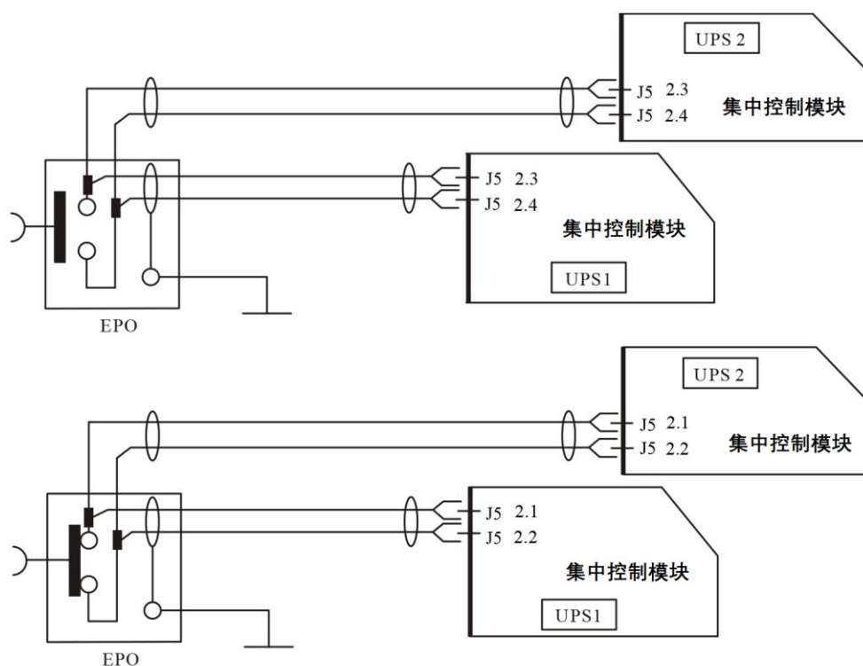
图 7-4 远程 EPO 电路连接图
