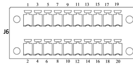
图 3-5 干接点接口 J6 示意图
