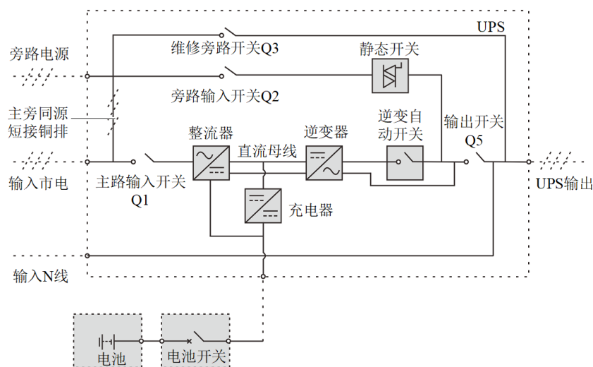
图 1-2 UPS 开关配置 (无开关、四开关)
