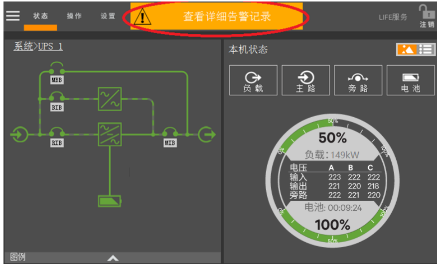
图 4-39 椭圆框中为状态条
