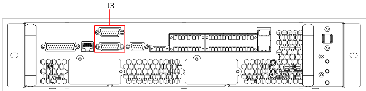
图 7-3 旁路模块并机接口 (J3) 图
