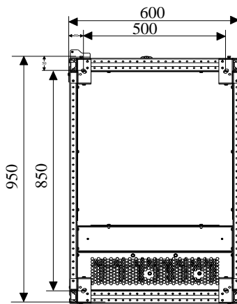
底视图
