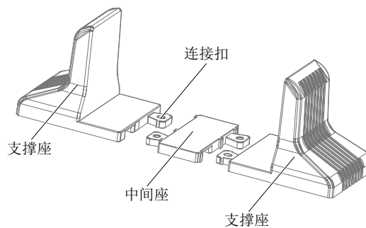
图2-5 连接支撑座和中间座
