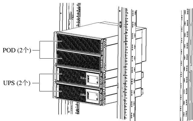
图3-1 1+1 并机系统安装示意图
