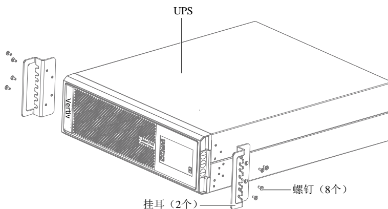
图2-7 安装挂耳
