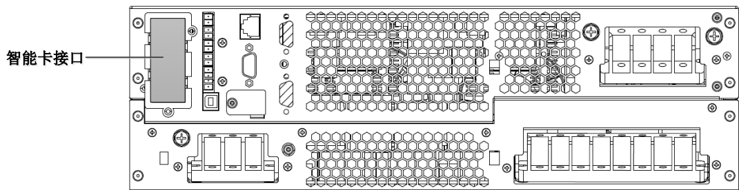
图6-1 智能卡安装示意图（后视图）
