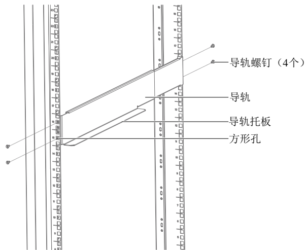
图2-10 安装导轨
