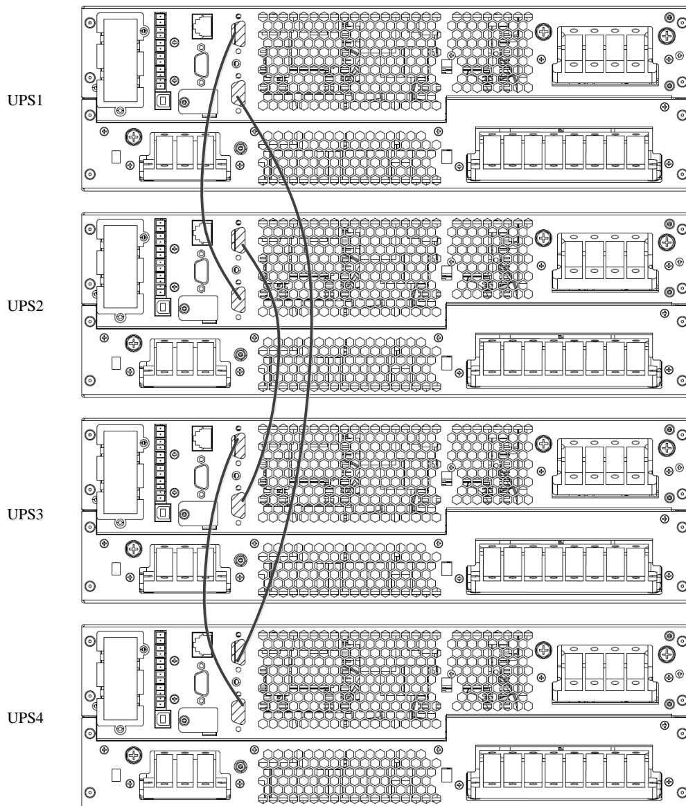
图3-3 3+1 并机电缆连接示意图
