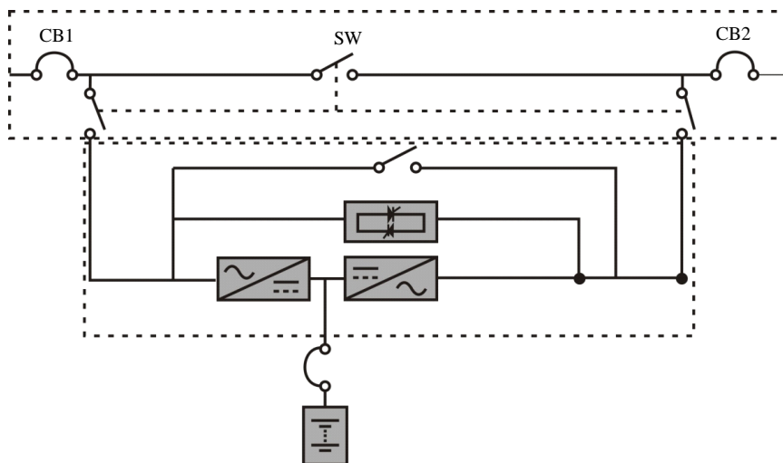
图5-9 带外部维修旁路的 UPS 单机配置示例
