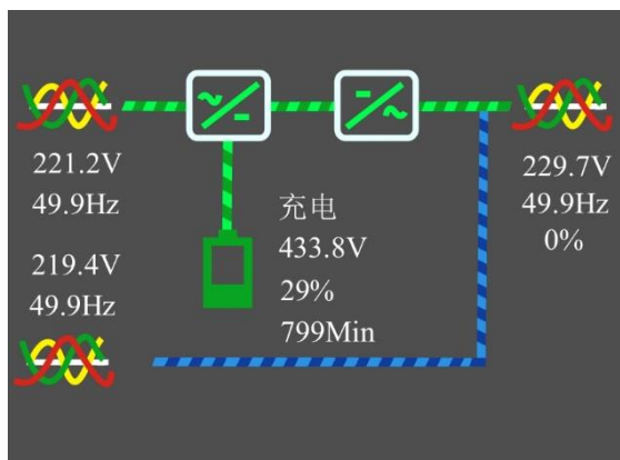
图4-11 流程图屏
