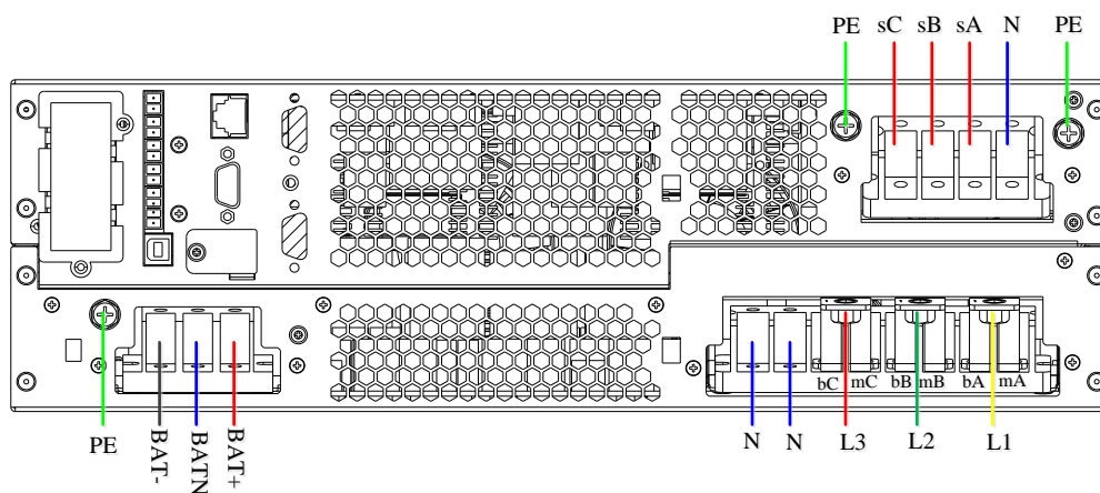
图2-14 接线示意图（三进三出，主旁同源）
