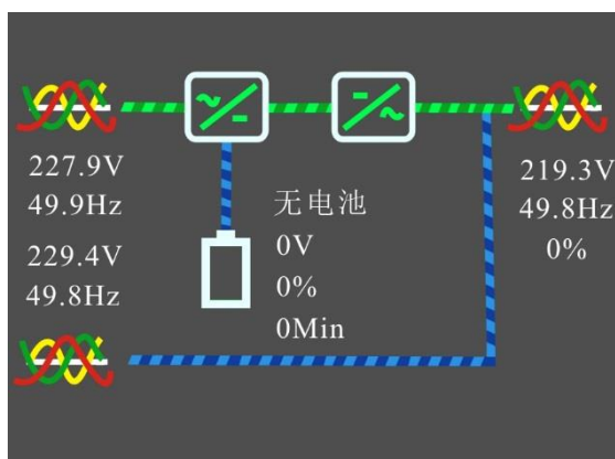
图5-5 旁路转逆变模式
