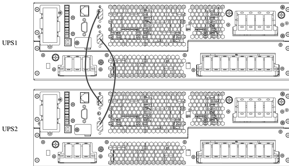
图3-9 LBS 电缆连接图
