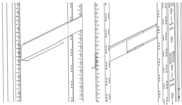
图2-11 导轨安装完成图
