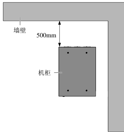
图2-3 操作空间示意图（机架式安装，顶视图）
