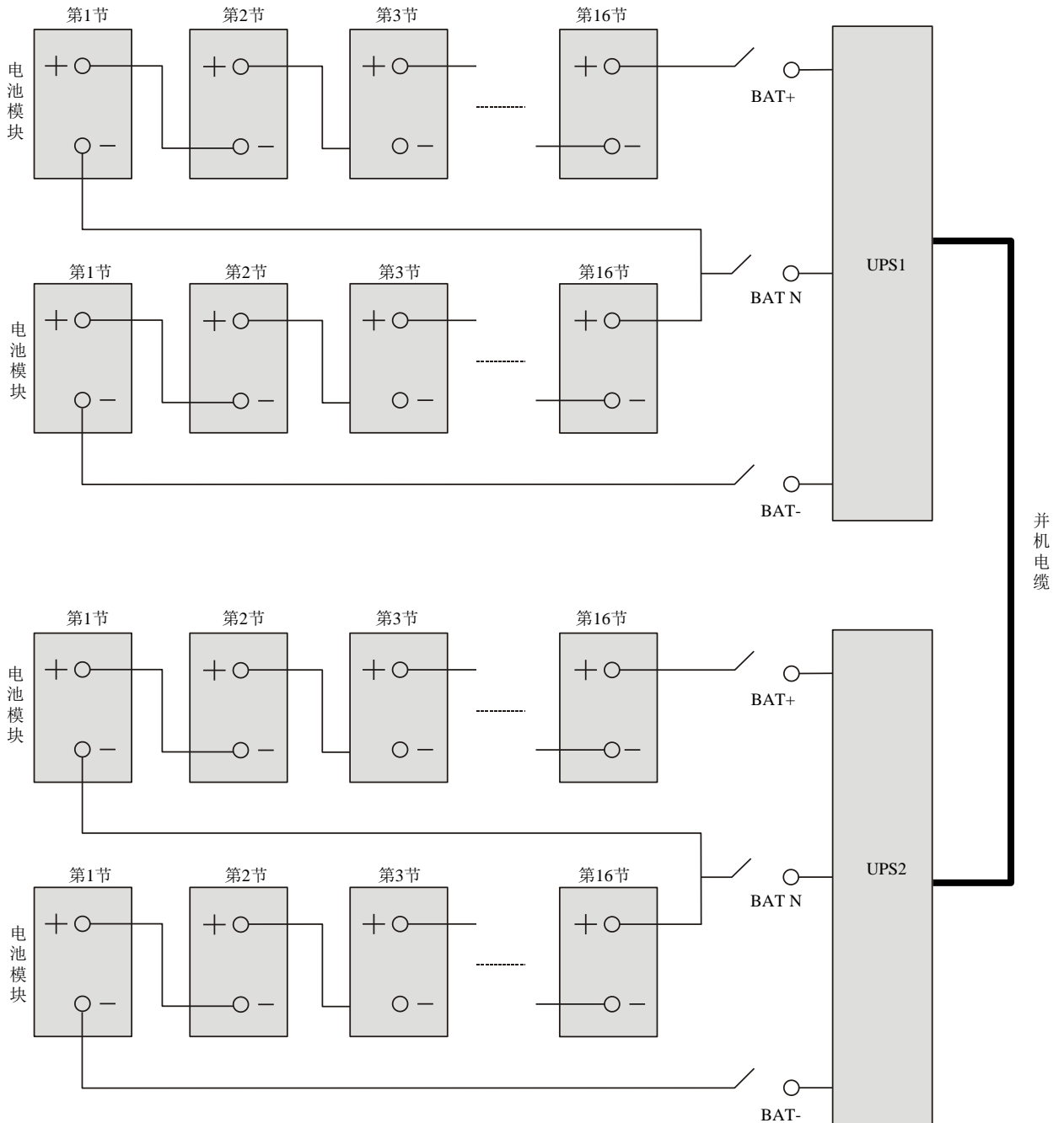
图3-4 30kVA 独立使用电池组接线原理图
