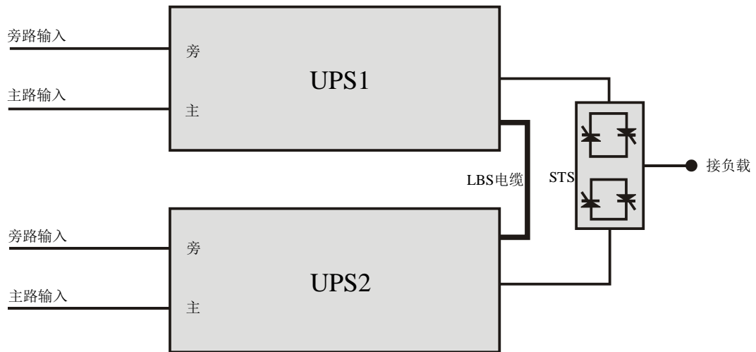
图3-8 LBS 系统示意图
