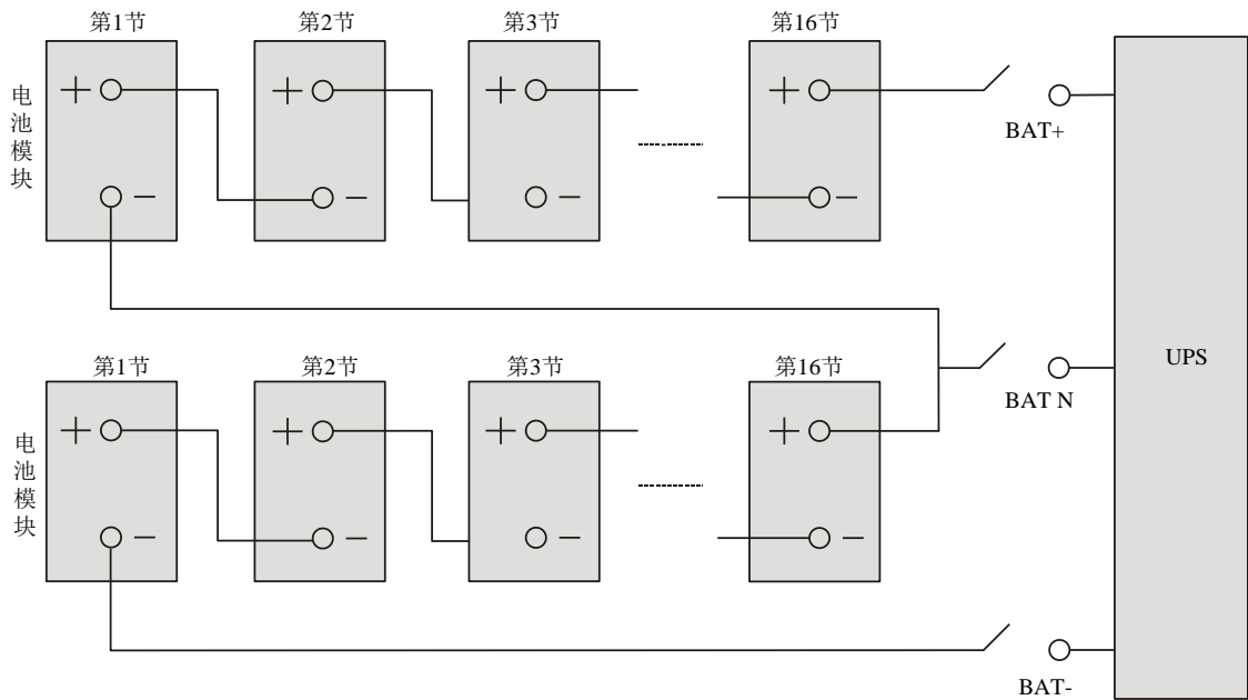
图2-17 电池组接线原理图
