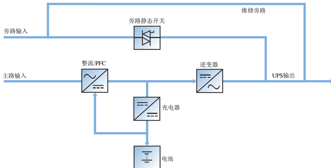
图1-4 UPS 工作原理
