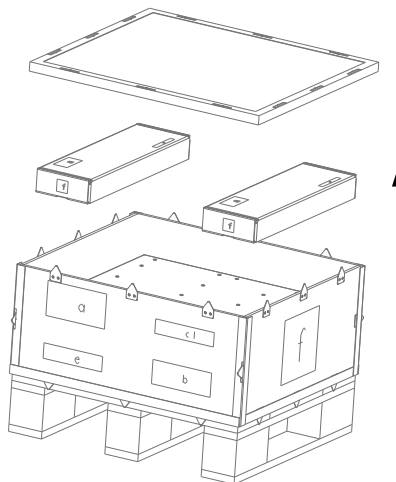
图2-2 开箱示意图
