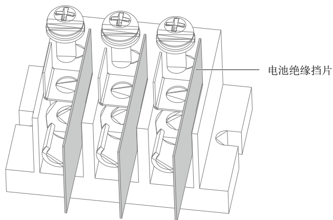
图2-16 安装电池绝缘挡片示意图
