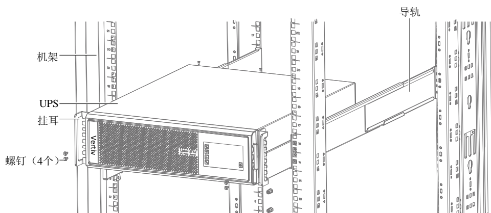
图2-12 安装 UPS
