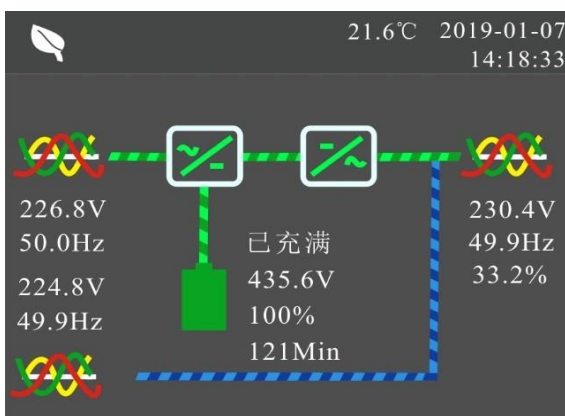
图5 流程图界面
