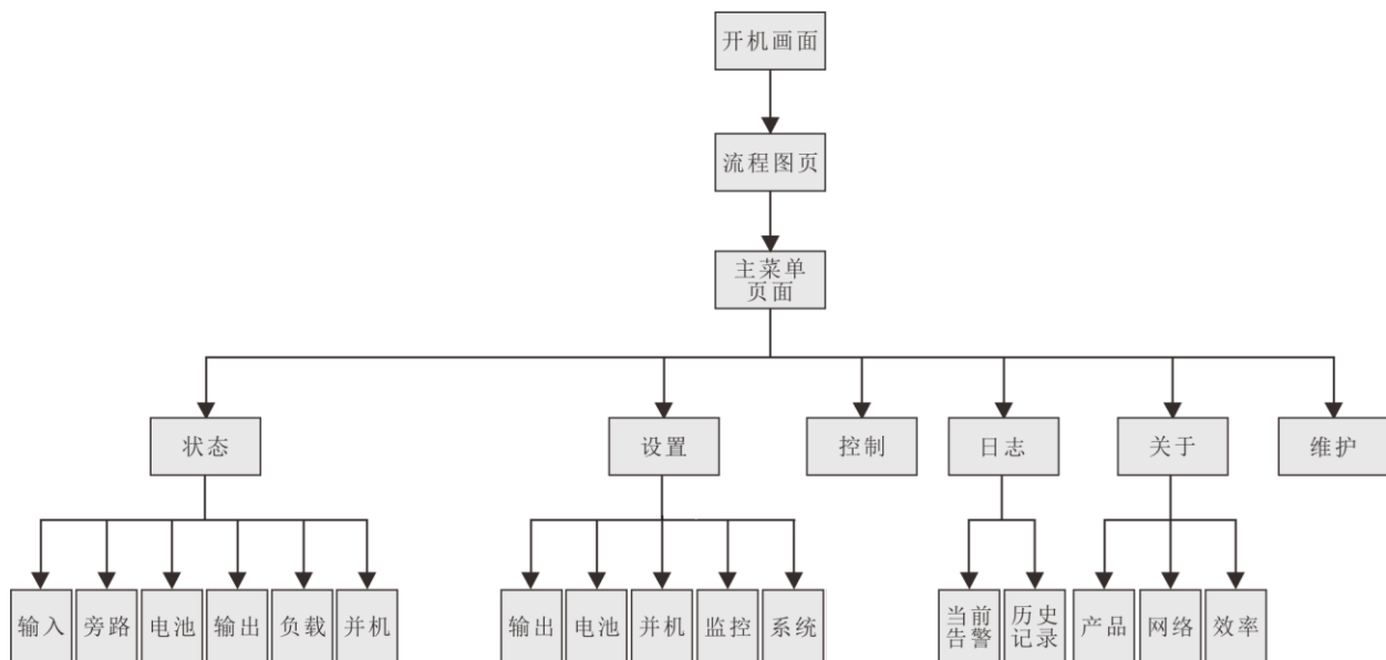
图4-9 菜单结构图
