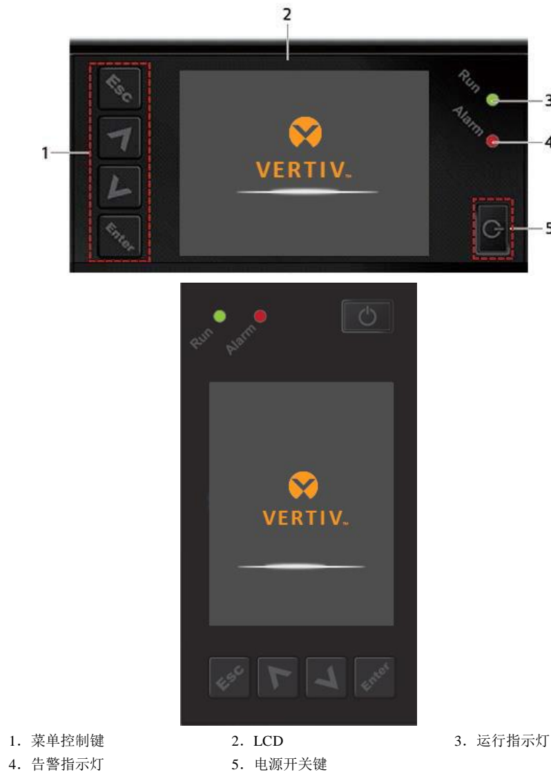
图4-1 操作显示面板
