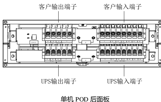
图8-1单机 POD 前面板和后面板
