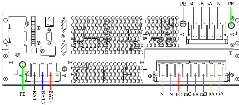
图2-15 三进三出，主旁不同源接线示意图
