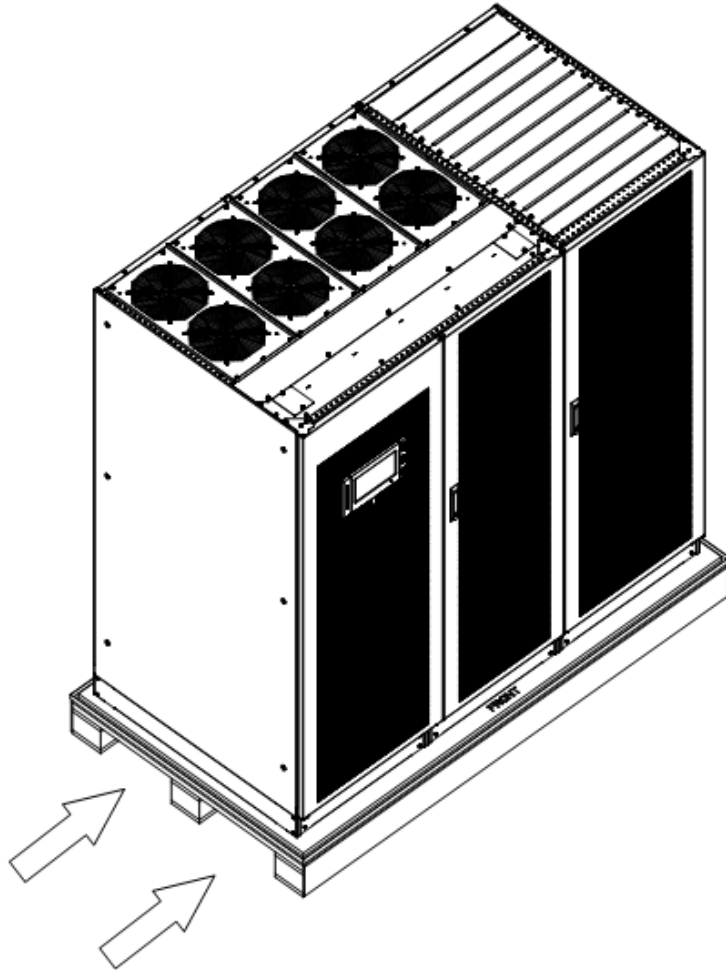
图 2-1 叉车叉入方向及运输示意图
