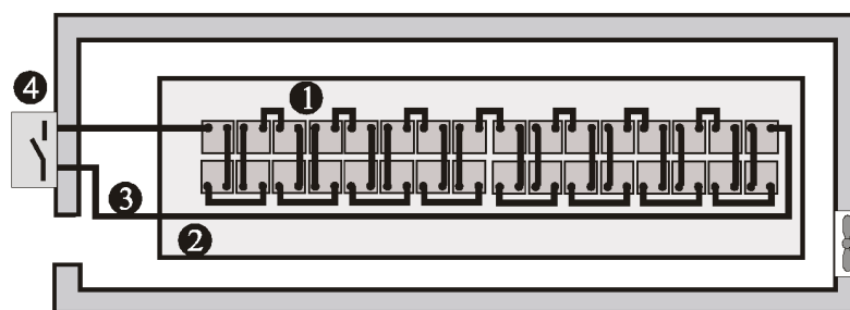
图 6-1 电池房设计
