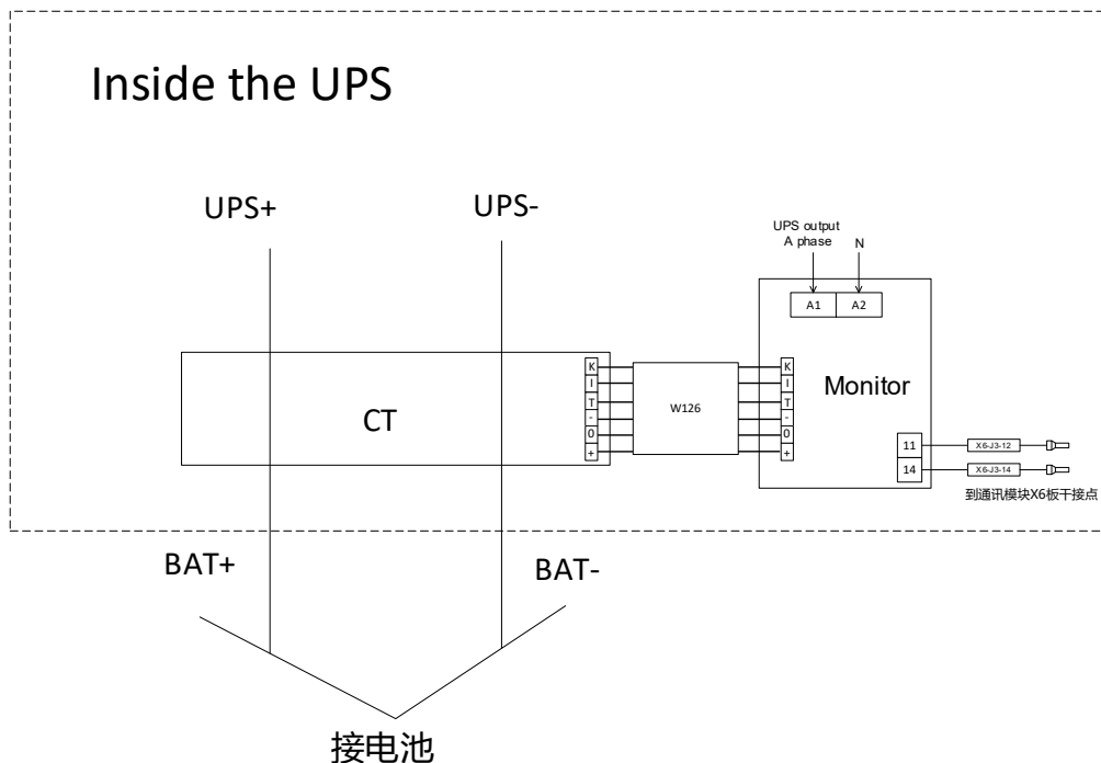
图 6-3 电池接地故障选件接线示意图
