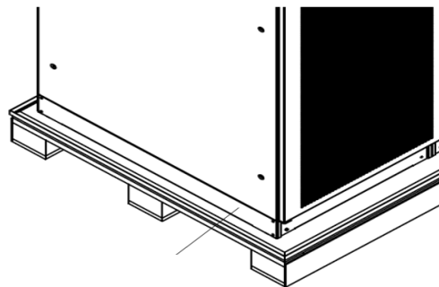
图 2-3 拆除防鼠挡板
