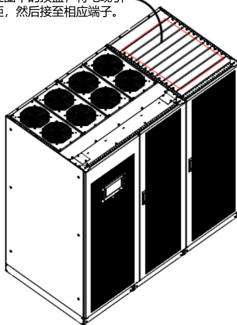
1250kVA 上进线
