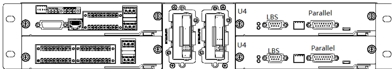
图 7-9 系统控制模块 LBS 接口和并机接口 (Parallel) 图
