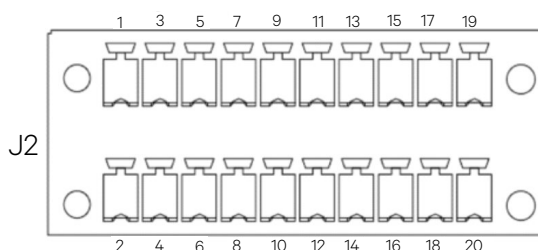
图 3-8 干接点接口 J2 示意图
