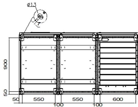
底视图
