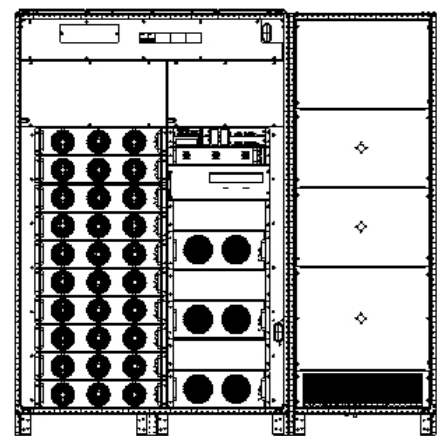
正视图 (门开)
