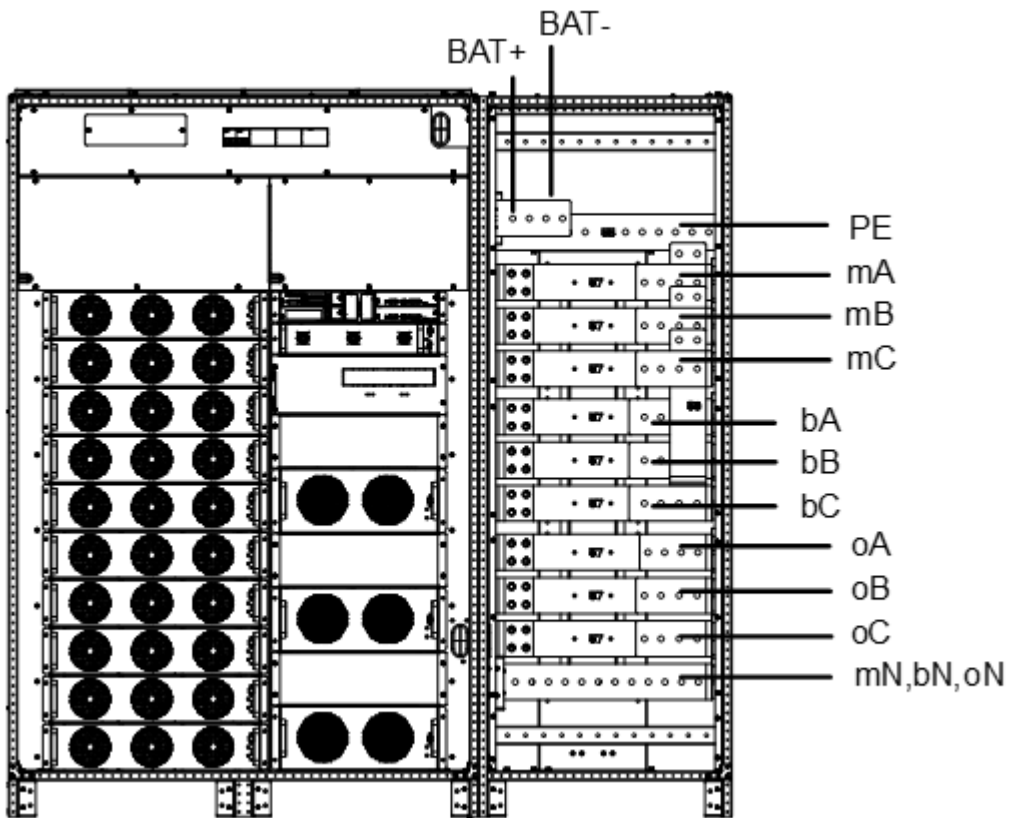
1250kVA 接线端子（无开关）
