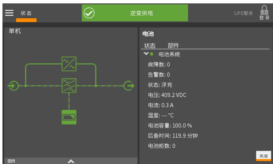
图 4-37 本机状态--电池详情
