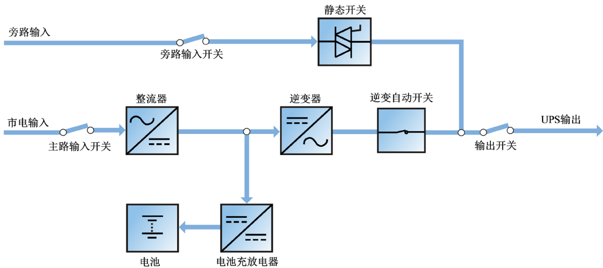
图 1-7 动态在线模式
