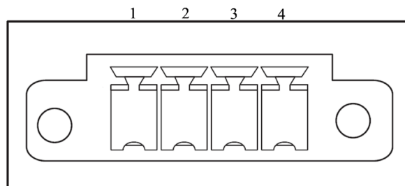
图 3-10 REPO 接口示意图
