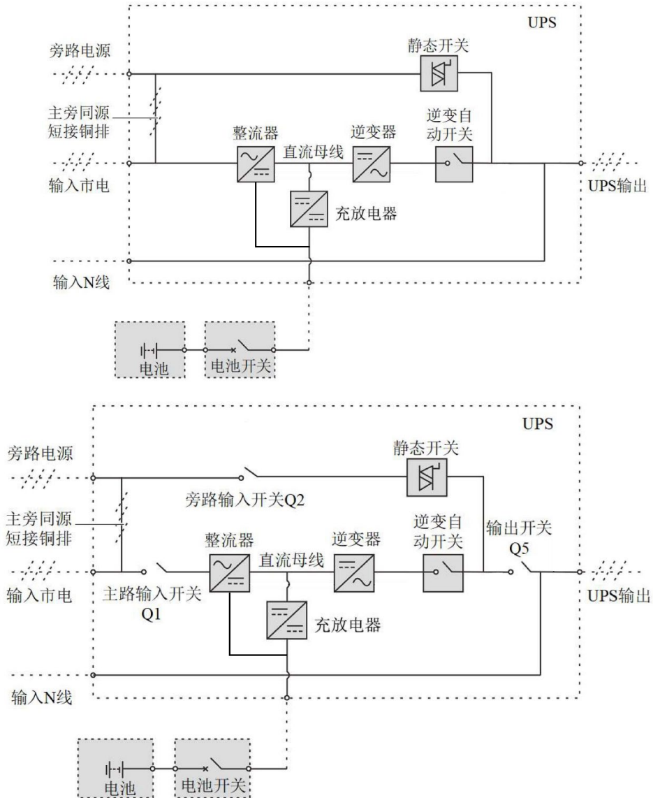
图 1-2 UPS 开关配置（无开关、三开关）
