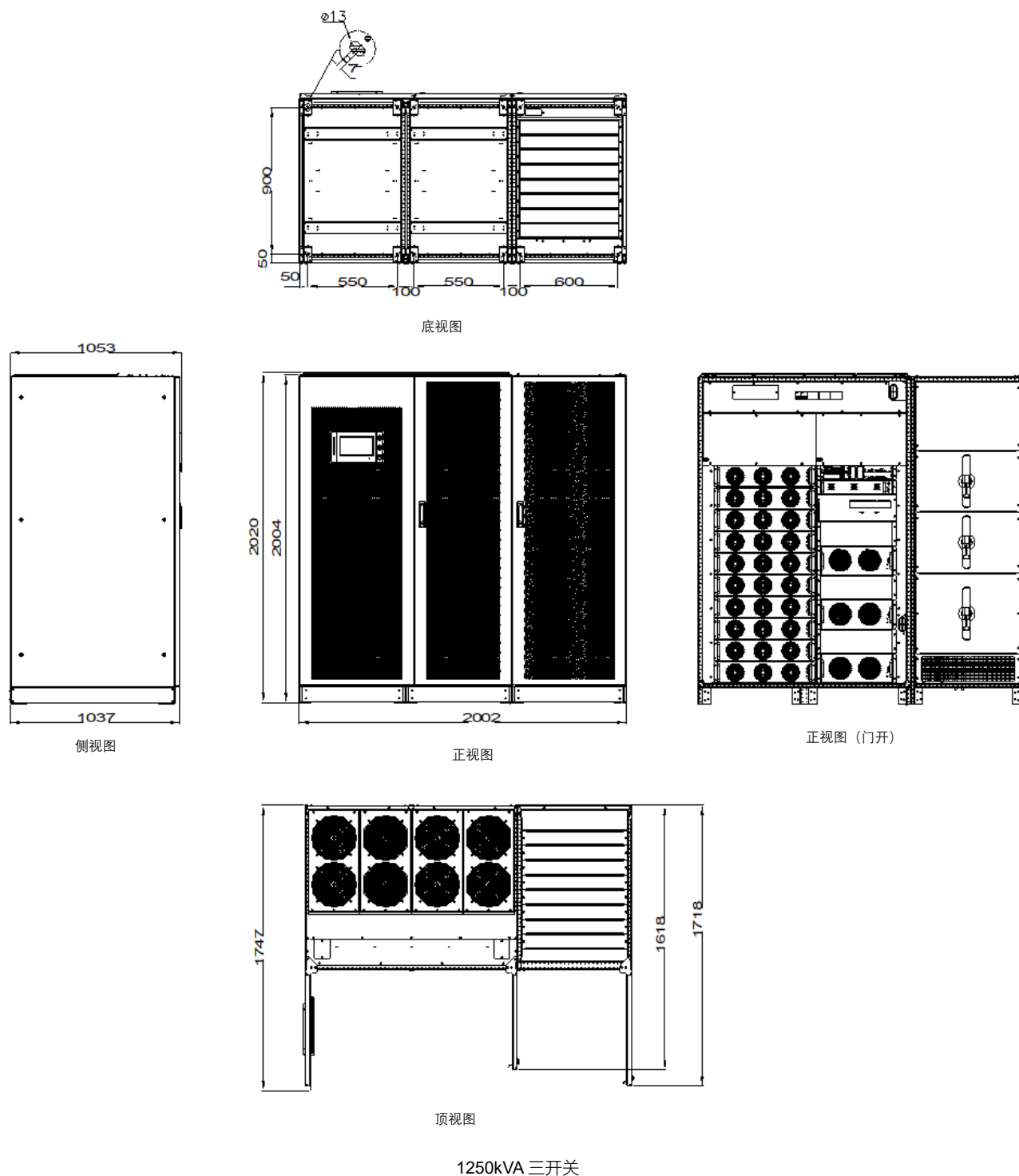
图 2-5 1250kVA 安装尺寸示意图 (单位: mm)
