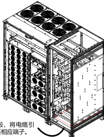
1250kVA 下进线
