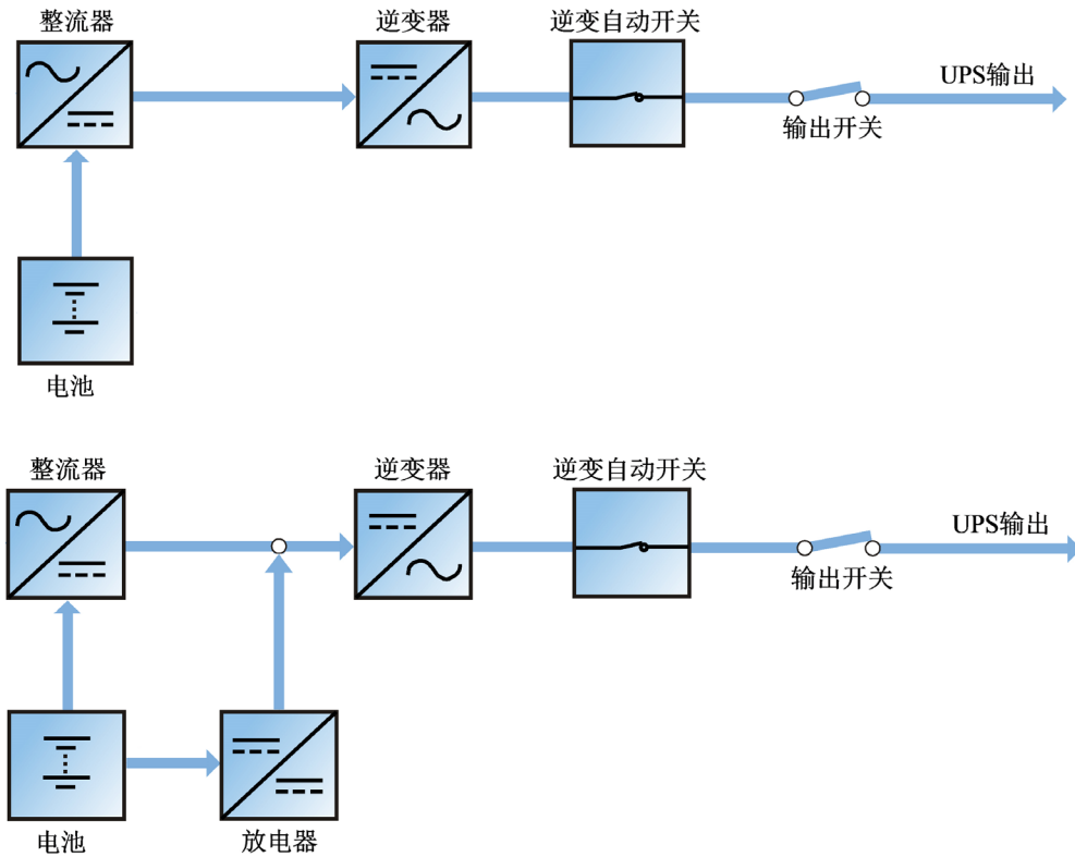
图 1-4 电池模式运行示意图
