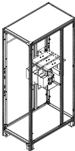
图 8-7 反灌保护柜选件安装示意图
