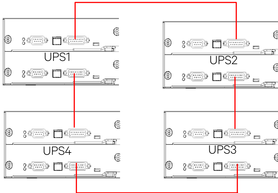
图 7-2 并机系统并机电缆连接
