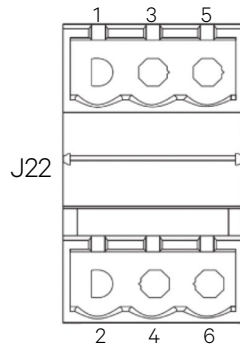
图 3-6 干接点接口 J22 示意图
