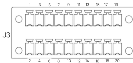
图 3-5 干接点接口 J3 示意图
