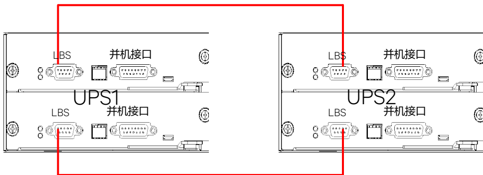
图 7-7 典型同步双母线系统的 LBS 电缆连接（单机）
