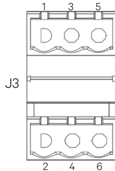
图 3-9 干接点接口 X7 J3 示意图
