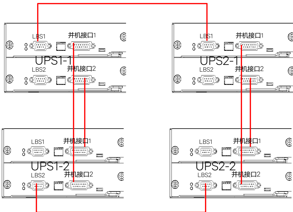
图 7-8 典型同步双母线系统的 LBS 电缆连接（并机）
