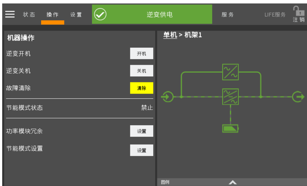
图 5-9 切换 UPS 至正常模式
