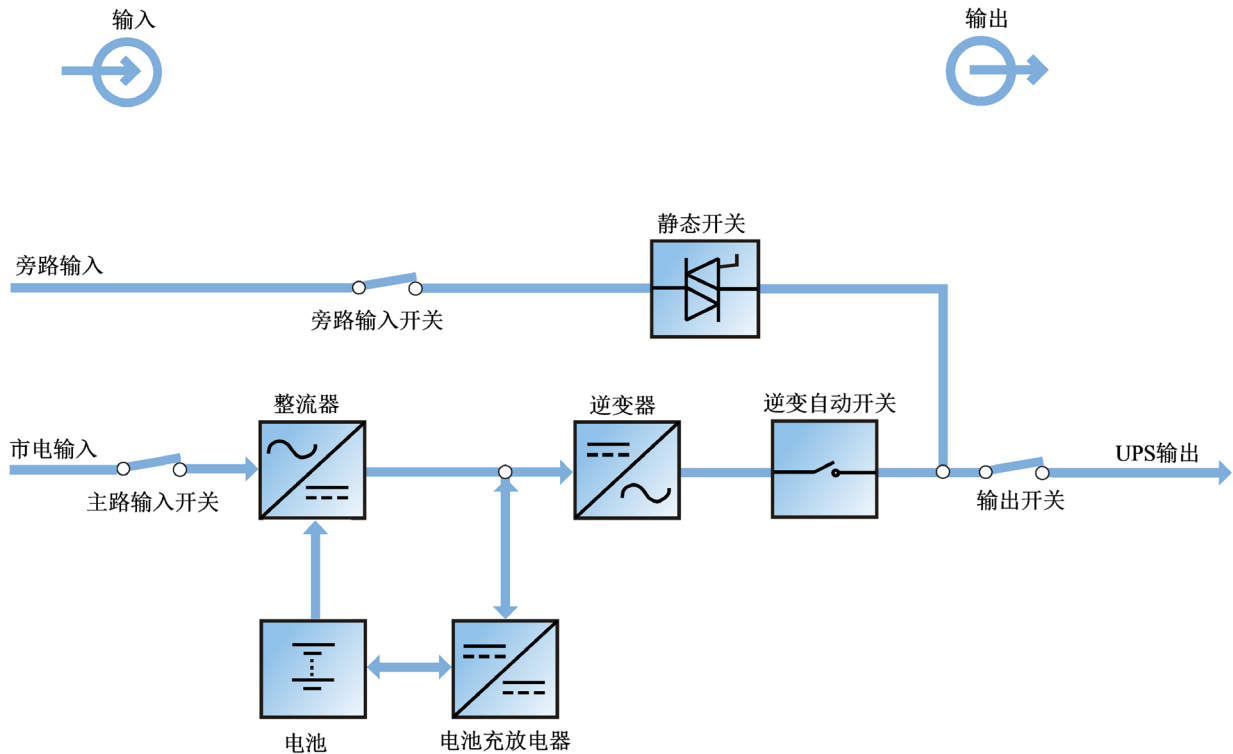
图1-1 UPS 单机工作原理框图（无开关、三开关）
