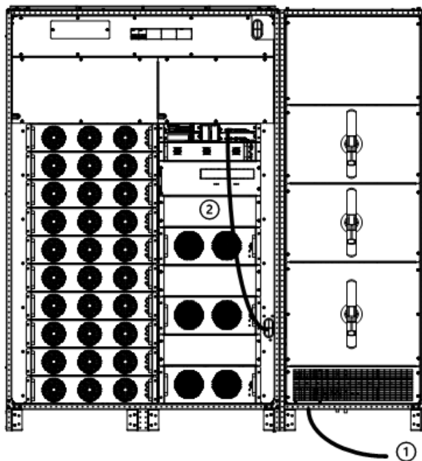
图 3-12 信号电缆走线示意图（下进线）
