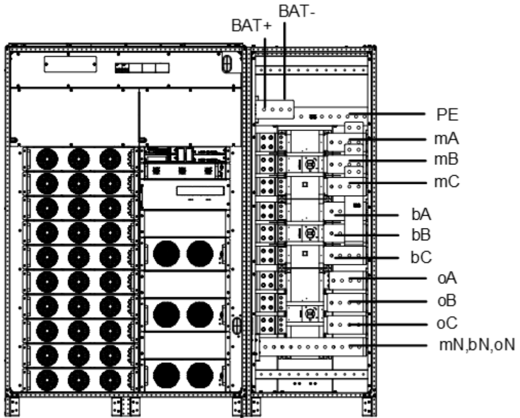
1250kVA 接线端子 (三开关)
