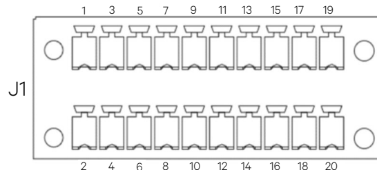
图 3-7 干接点接口 J1 示意图
