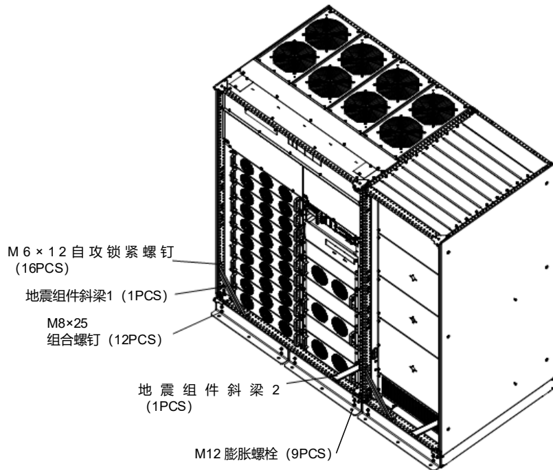
图 8-2 地震选件安装示意图（正面安装）
