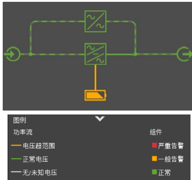
图 4-6 模拟显示，正常模式运行
