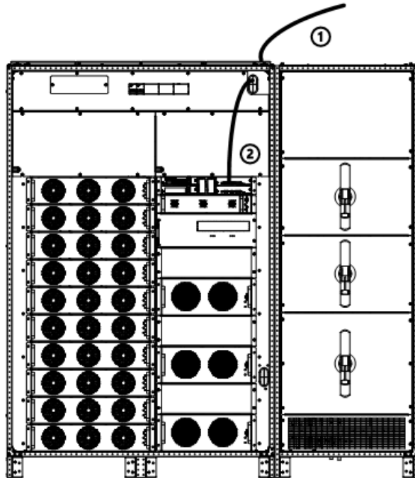
图 3-11 信号电缆走线示意图（上进线）
