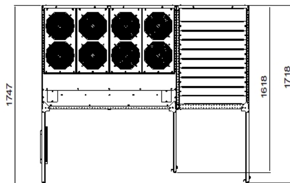
正视图
