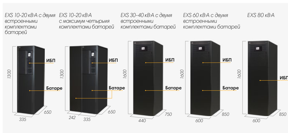
Архитектура Liebert EXS
