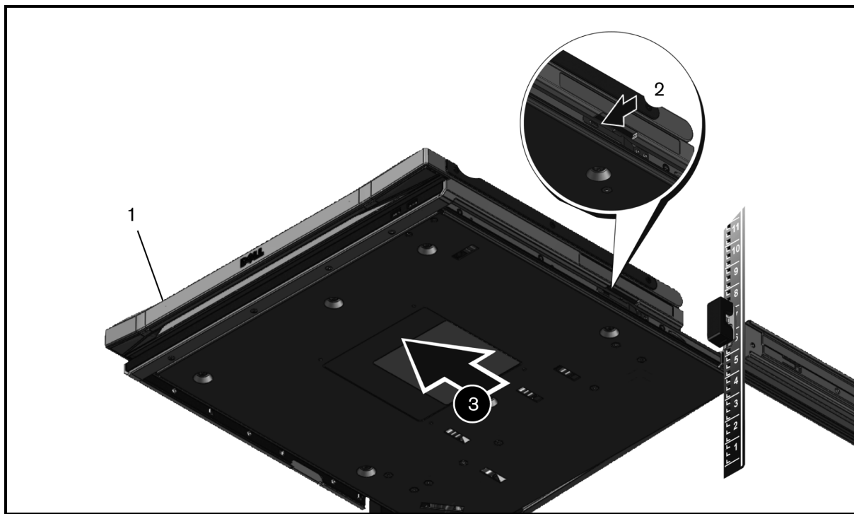
図 4.1 コンソール・トレイのラックからの取り外し
