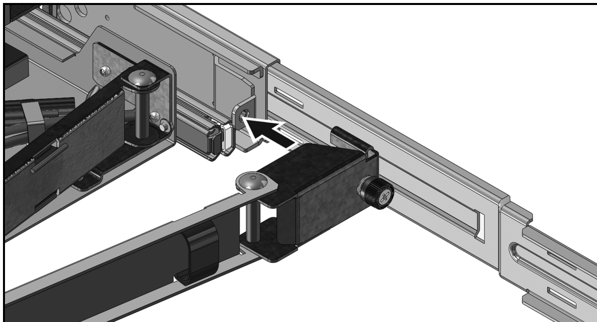
図 2.6 ケーブル管理アーム(CMA)の取り付け
