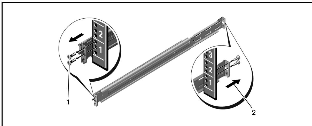
Figura 4.3 Extracción de los carriles con herramientas
